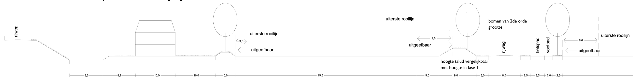
Profiel 3: doorsnede over de zone tussen de Maasdijk en de centrale ontsluitingsweg
