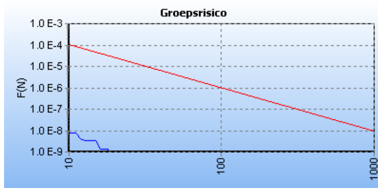
Figuur 5.4 FN curve voor N-528-50 van N.V. Nederlandse Gasunie voor de kilometer tussen stationing 0.00 en stationing 1000.00
