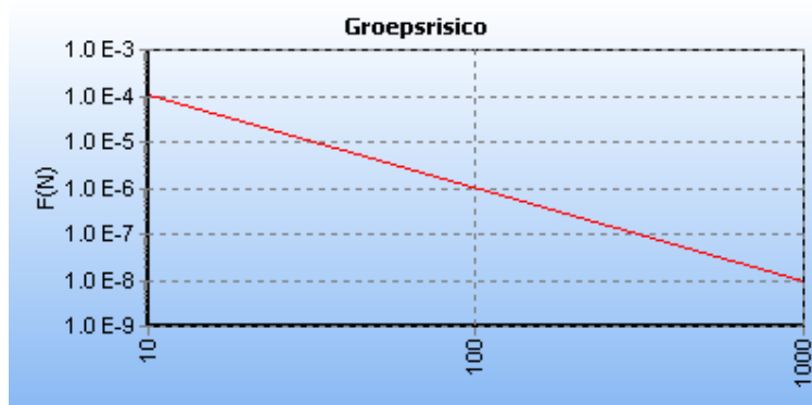
Figuur 5.6 FN curve voor N-528-57 van N.V. Nederlandse Gasunie voor de kilometer tussen stationing 0.00 en stationing 1000.00
