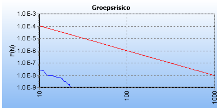
Figuur 5.8 FN curve voor N-528-79 van N.V. Nederlandse Gasunie voor de kilometer tussen stationing 0.00 en stationing 50.00
