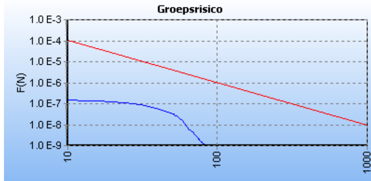
Figuur 5.1 FN curve voor A-670 van N.V. Nederlandse Gasunie voor de kilometer tussen stationing 20940.00 en stationing 21940.00
