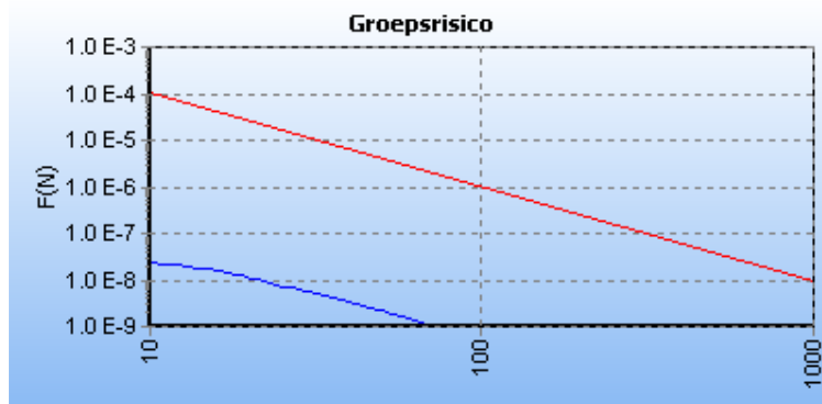
Figuur 5.2 FN curve voor A-646 van N.V. Nederlandse Gasunie voor de kilometer tussen stationing 20770.00 en stationing 21770.00
