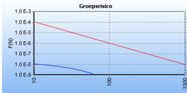
Figuur 5.9 FN curve voor Enschede 24in van Zebra Gasnetwerk BV voor de kilometer tussen stationing 0.00 en stationing 1000.00
