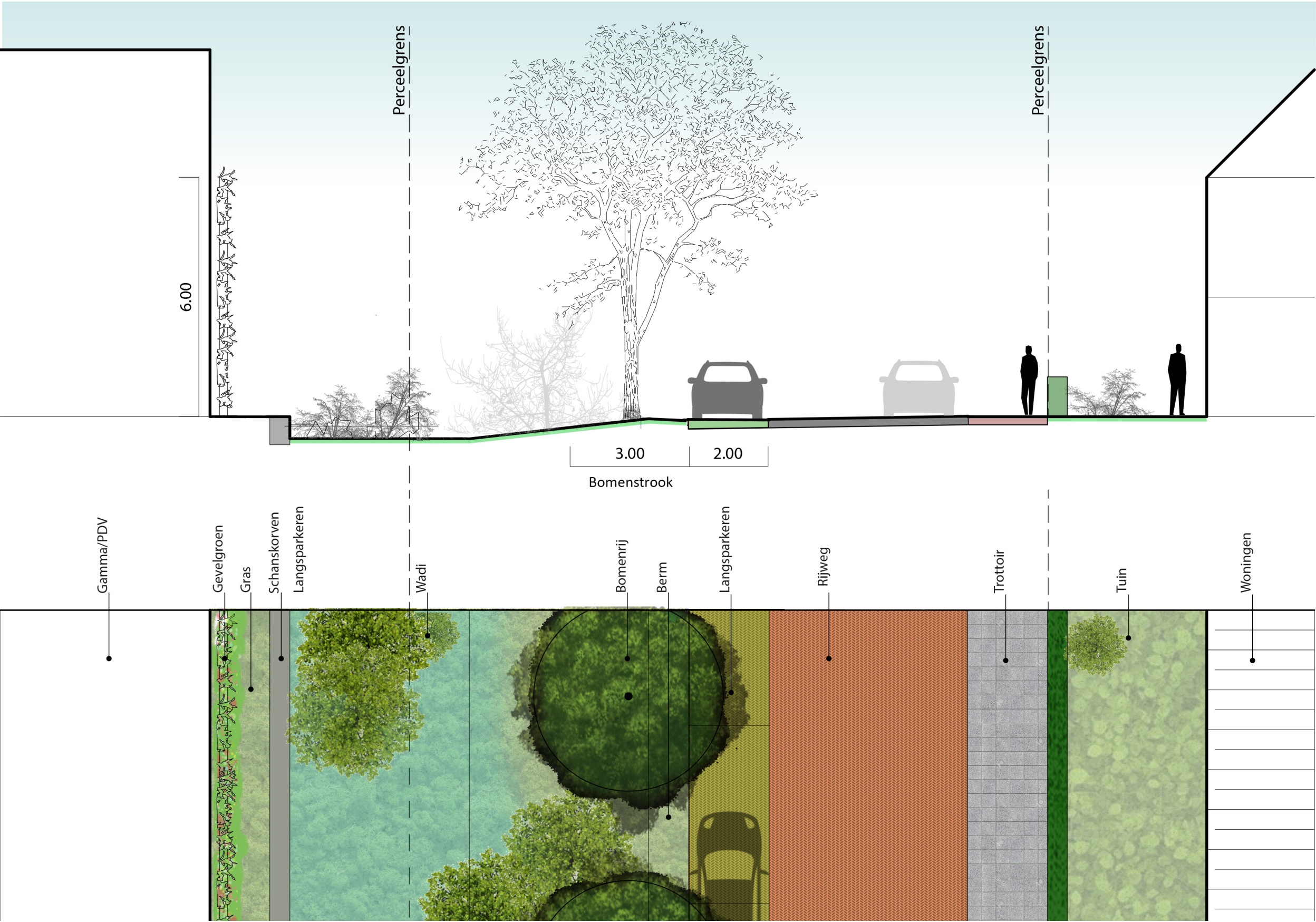
Principeprofiel wadi
