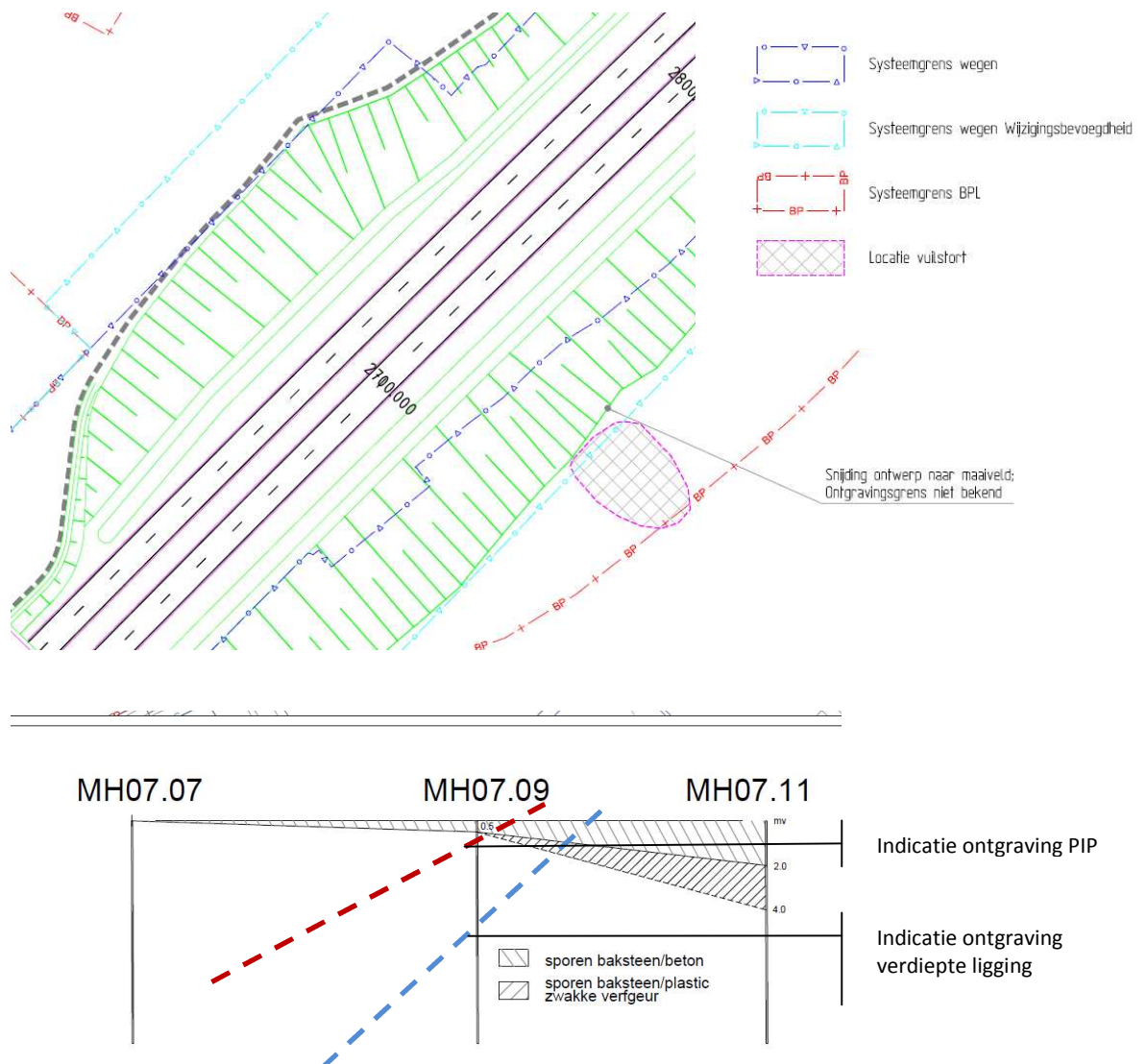
Figuur 5.2 Situatietekening stort Vaesrade
