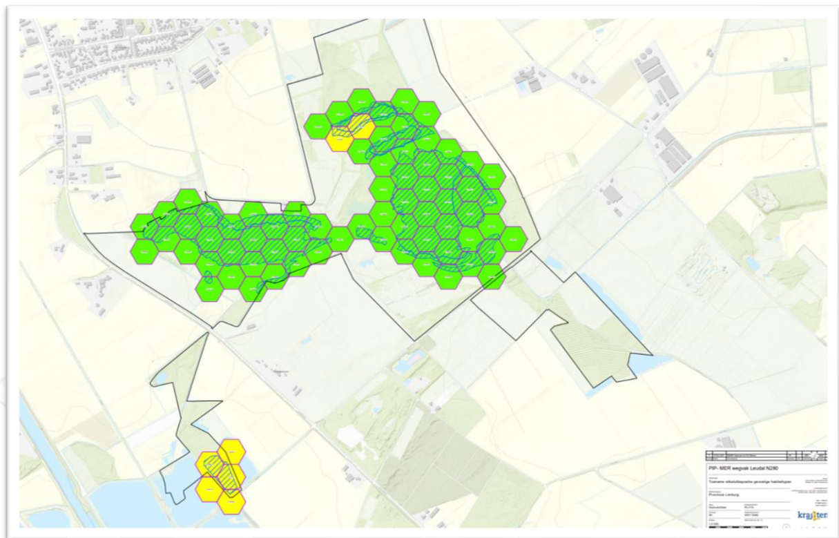
Figuur 11: Verspreidingskaart stikstofdepositie gebruiksfase Sarsven en De Banen (groen = geen toename; geel = toename)
