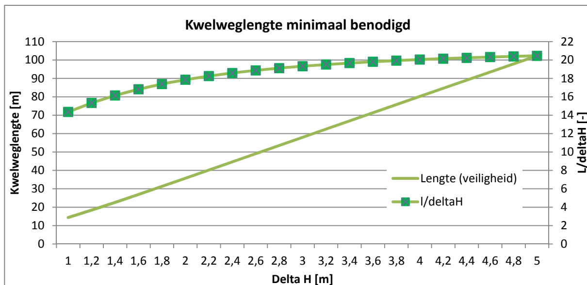
Figuur 2: De minimaal benodigde kwelweglengte in relatie tot het kritieke verval
