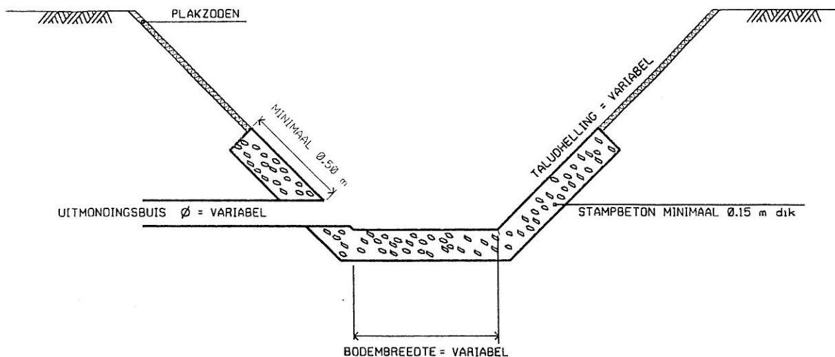
DWARSDOORSNEDE
