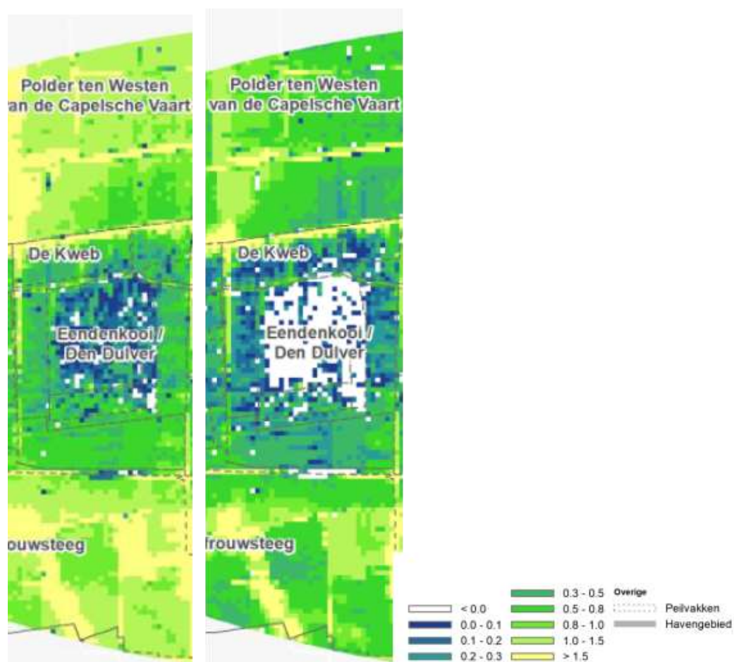
Figuur 3.6: De GLG (links) en GHG (rechts in en rondom de Den Dülver). Schaal legenda in cm -mv. Wit duidt op permanent water en van donkerblauw naar middelblauw verloopt de wegzakking tot 20 cm -mv.
