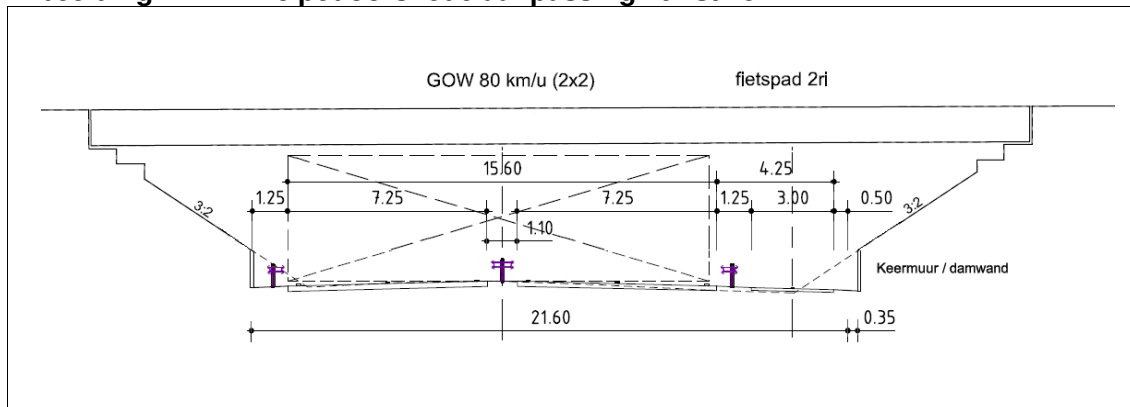
Afbeelding 7.1. Principeddoorsnede aanpassing kunstwerk A17
