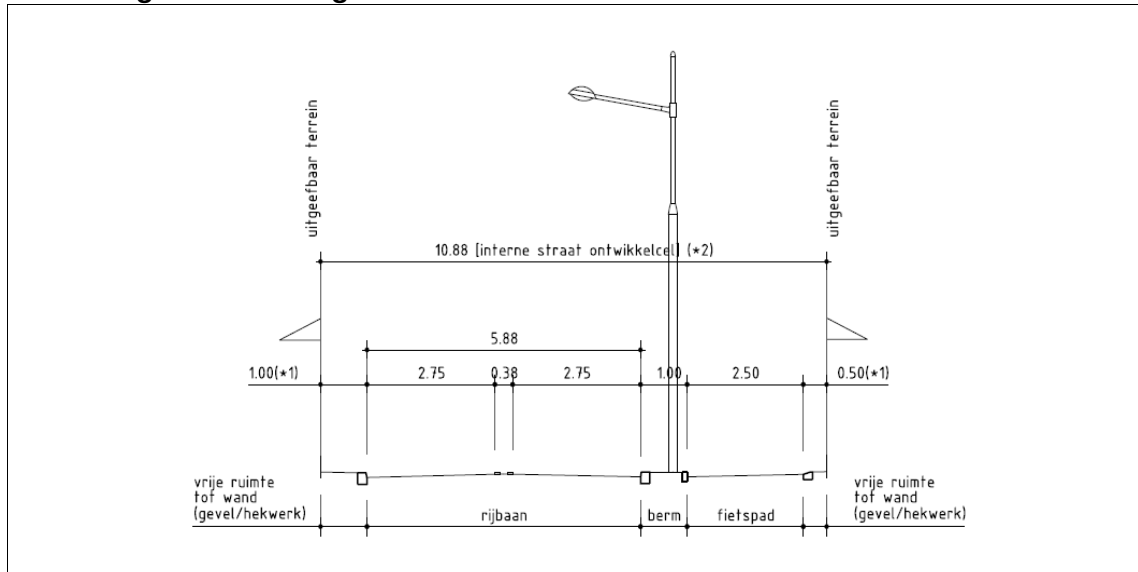
Abbeelding 5.2. Inrichting interne straat ontwikkelcellen
