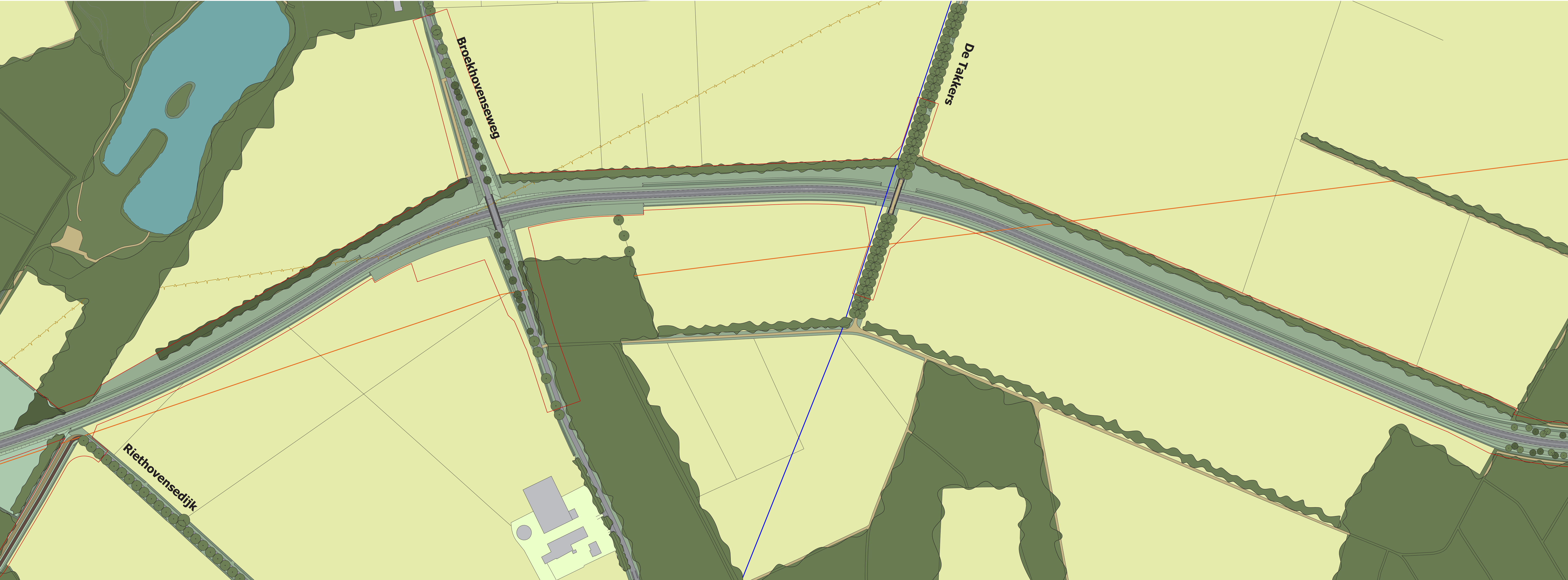
INRICHTINGSPLAN N69 - BLAD 2; SCHAAL 1:2.000
