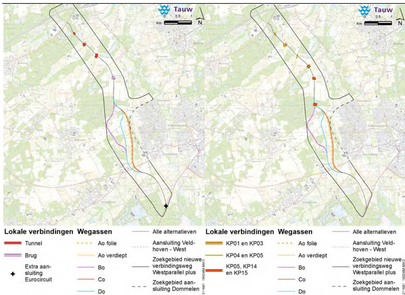
Figuur 9.10 Varianten lokale verbindingen (tunnels in plaats van bruggen, links en zoeken naar combinaties, rechts)
