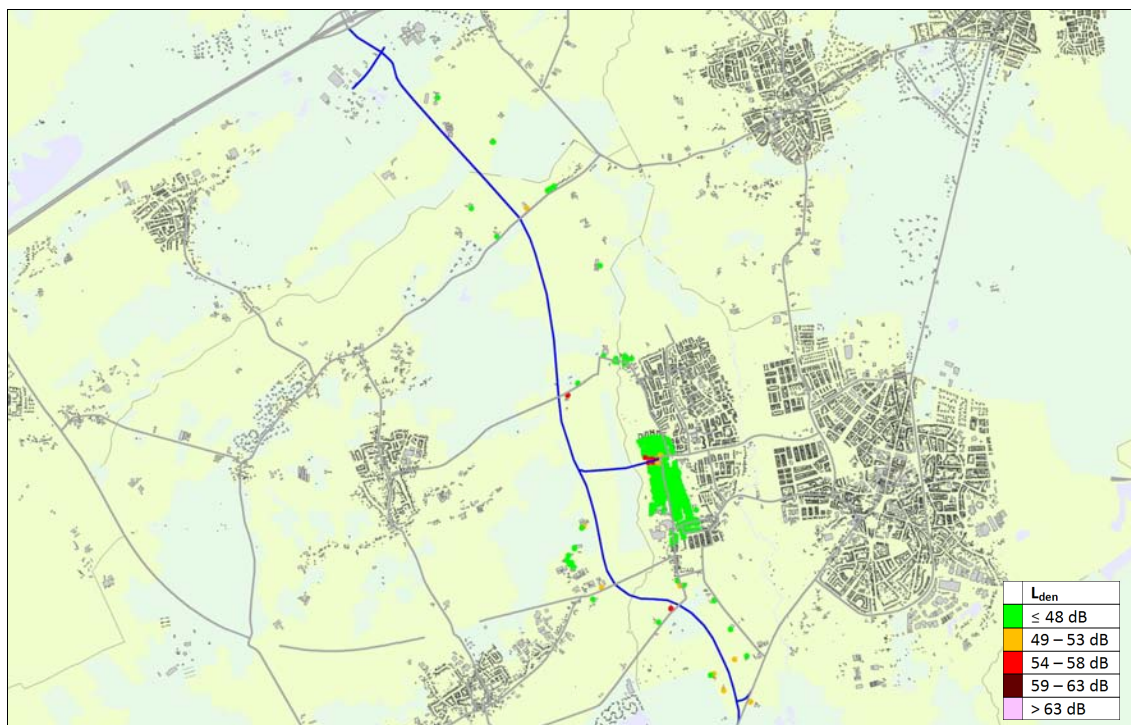
Figuur 6.5: Geluidsbelastingen ten gevolge van variant D1
