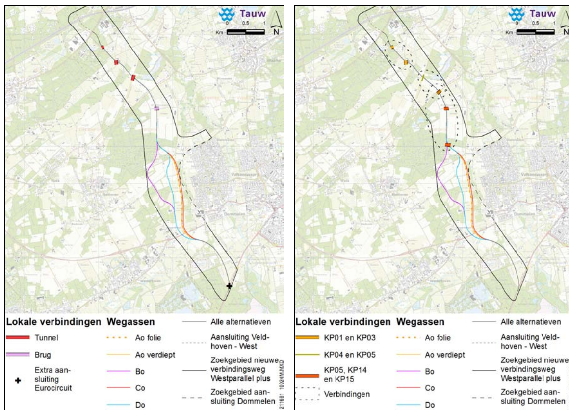
Figuur 9.19: Varianten lokale verbindingen (tunnels in plaats van bruggen, links en zoeken naar combinaties, rechts)
