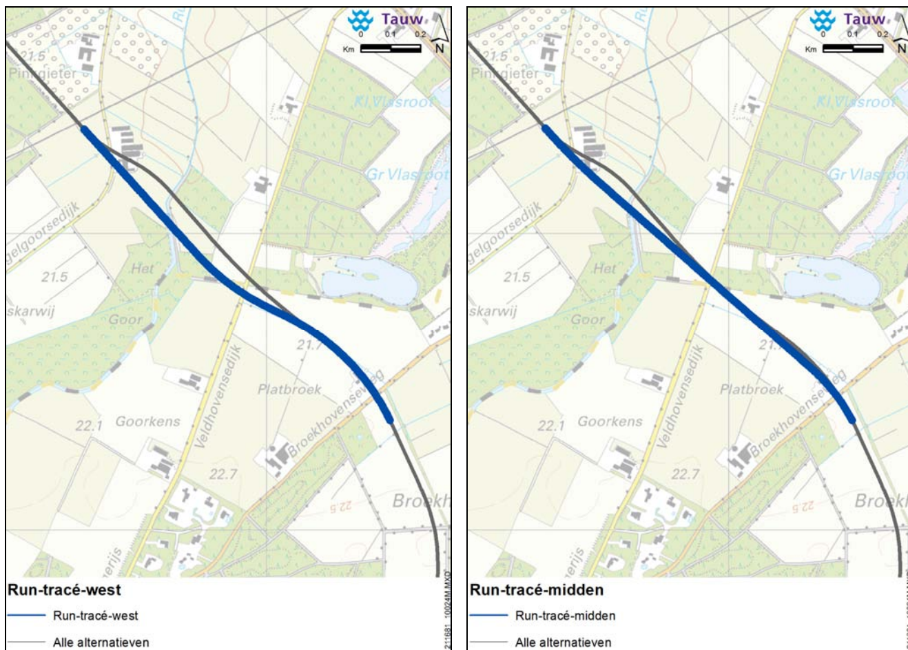
Figuur 9.17: Twee varianten met een meer westelijk trace nabij de Run voor alle vijf de alternatieven (midden/west)
