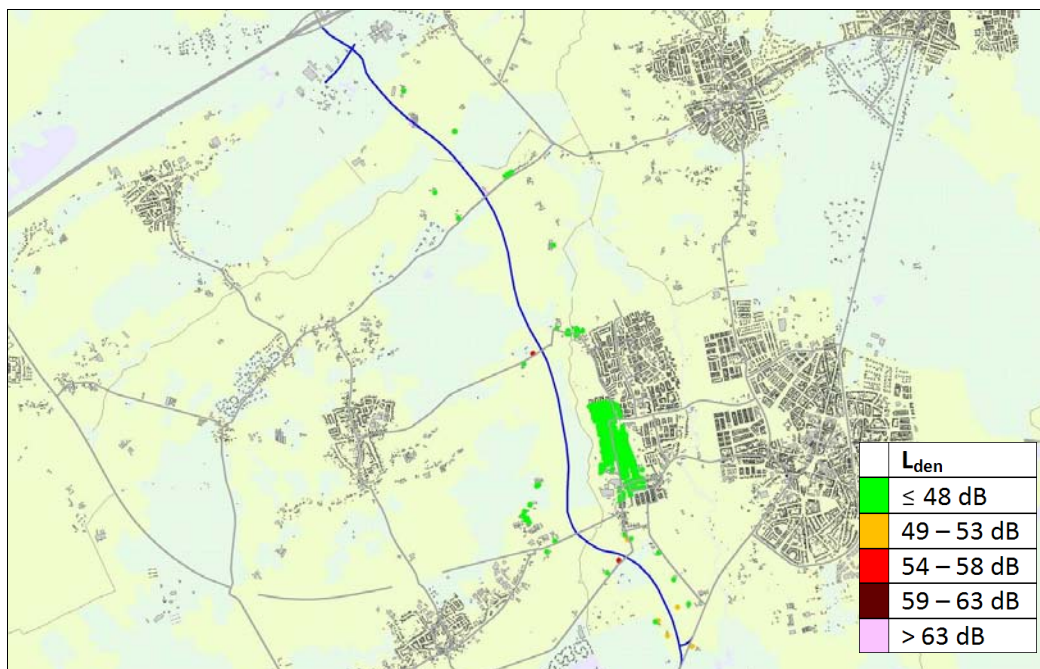
Figuur 5.3: Geluidsbelastingen alternatief A ten gevolge van de nieuwe weg
