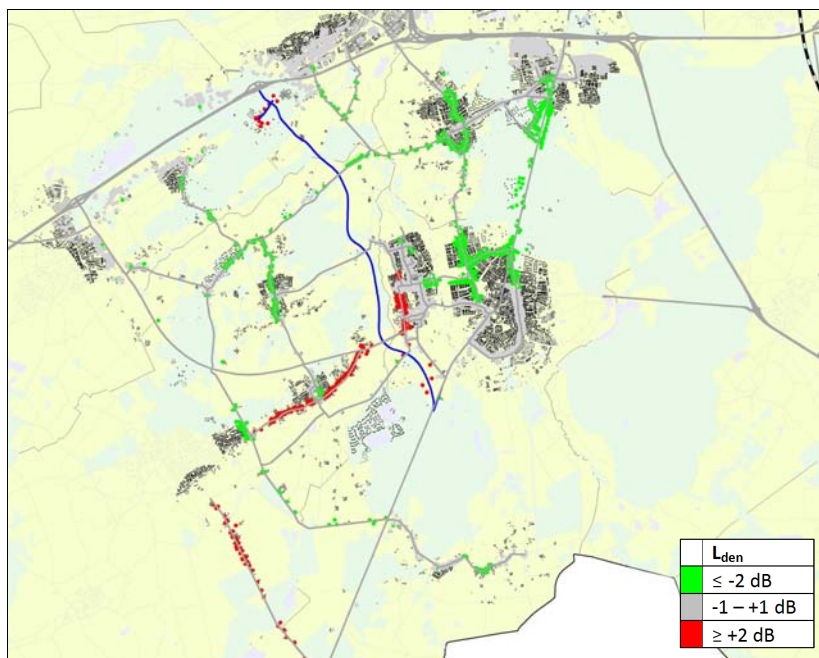
Figuur 9.7: Waarneembare geluidsverschillen Co t.o.v referentie
