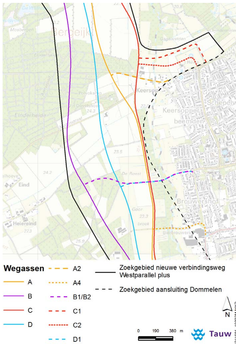
Figuur 6.3: Overzicht van de ligging van de 4 alternatieven en de bijbehorende zeven aansluitingsvarianten bij Dommelen
