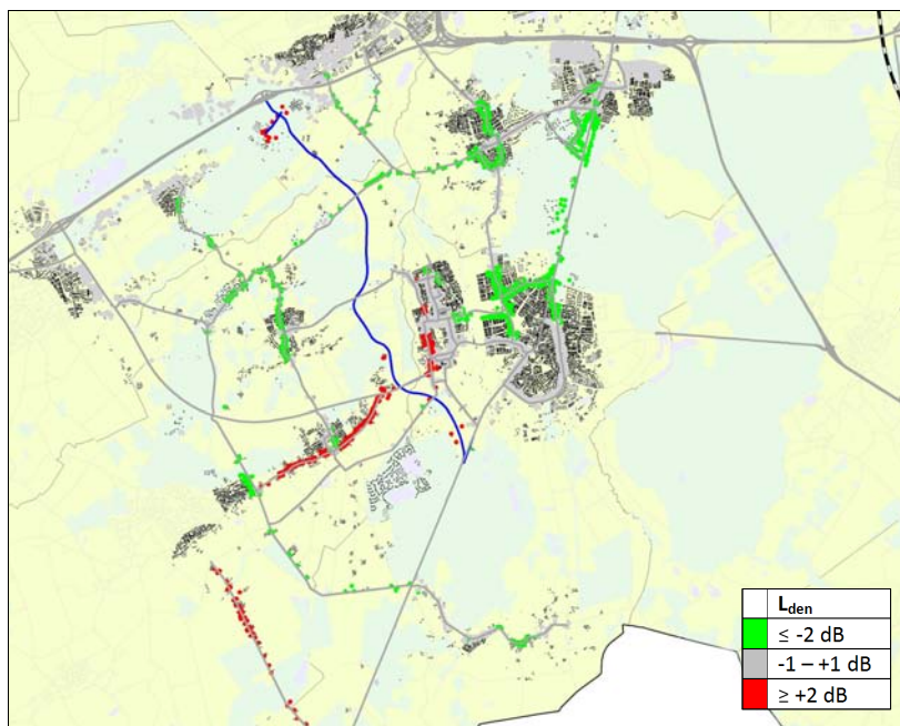
Figuur 9.6: Waarneembare geluidsverschillen Bo t.o.v referentie
