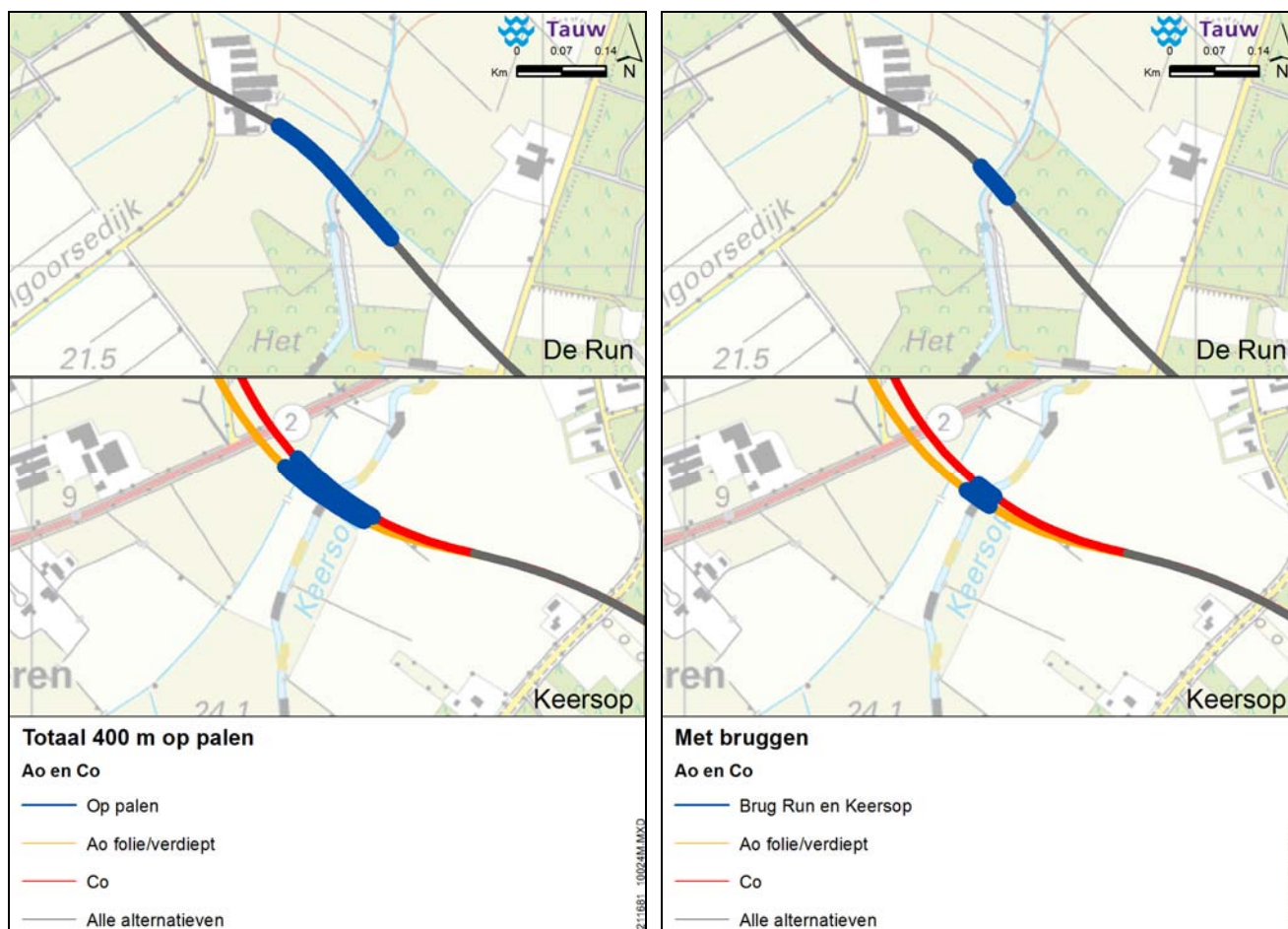
Figuur 9.16: Variant 400m op palen, respectievelijk 250 m (Run) en 150 m (Keersop) en variant met bruggen over de Run en de Keersop voor de alternatieven Ao-folie, Ao-verdiept en Co.
