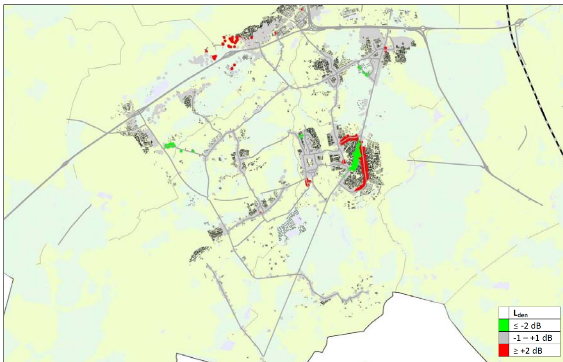
Figuur 4.1: Locaties waar sprake is van een waarneembare toe- of afname van de geluidsbelasting
