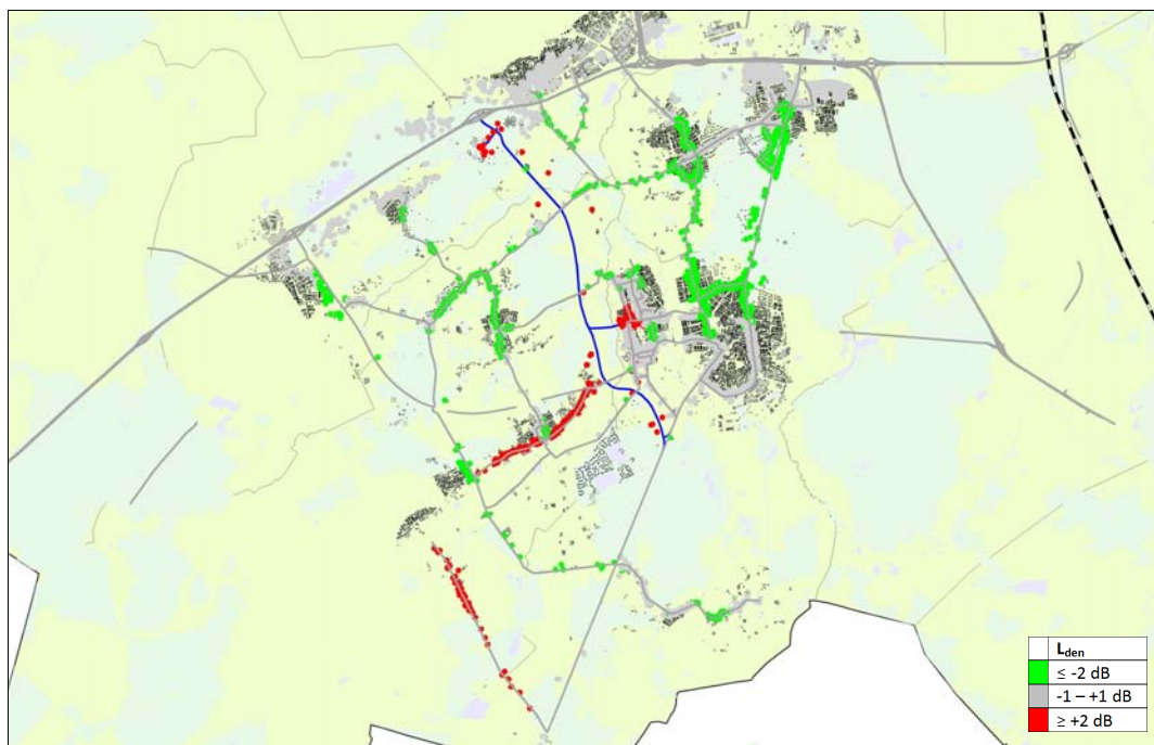
Figuur 6.3: Waarneembare geluidseffecten variant C2 ten opzichte van de referentie
