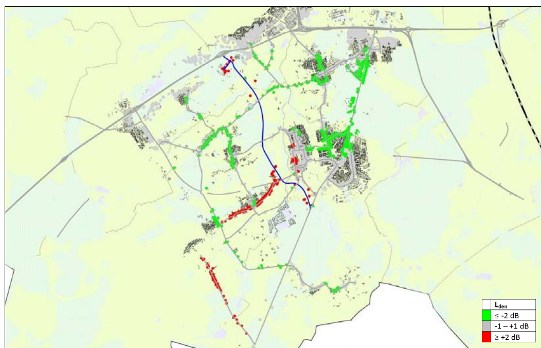
Figuur 5.2: Waarneembare geluidseffecten alternatief B ten opzichte van de referentie
