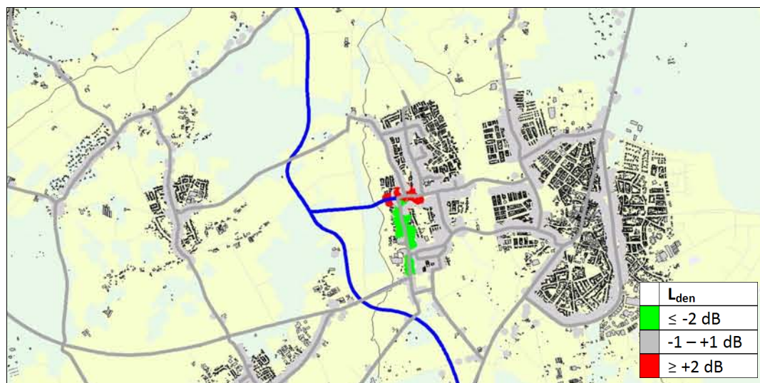
Figuur 9.11: Waarneembare toe- en afnamen van een extra midden-aansluiting voor alternatief Bo
