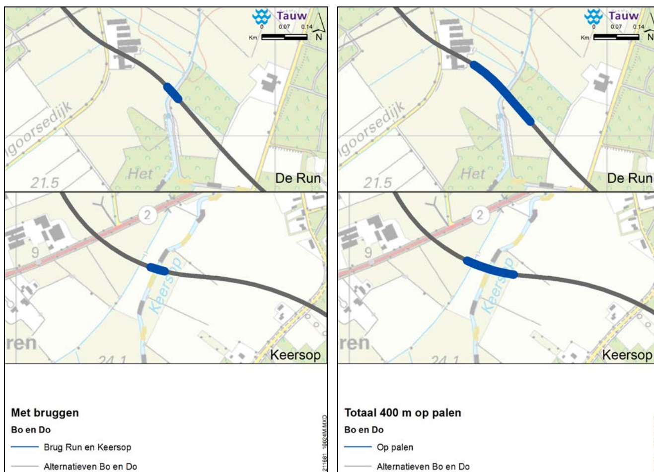
Figuur 9.15: Variant 400m op palen, respectievelijk 250 m (Run) en 150 m (Keersop) en variant met bruggen over de Run en de Keersop voor de alternatieven Bo en Do
