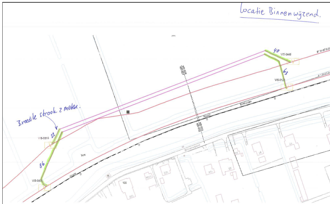
Afb. 2. Ligging van de leidingsleuven met afmetingen (aangeleverd 26 maart 2013)
