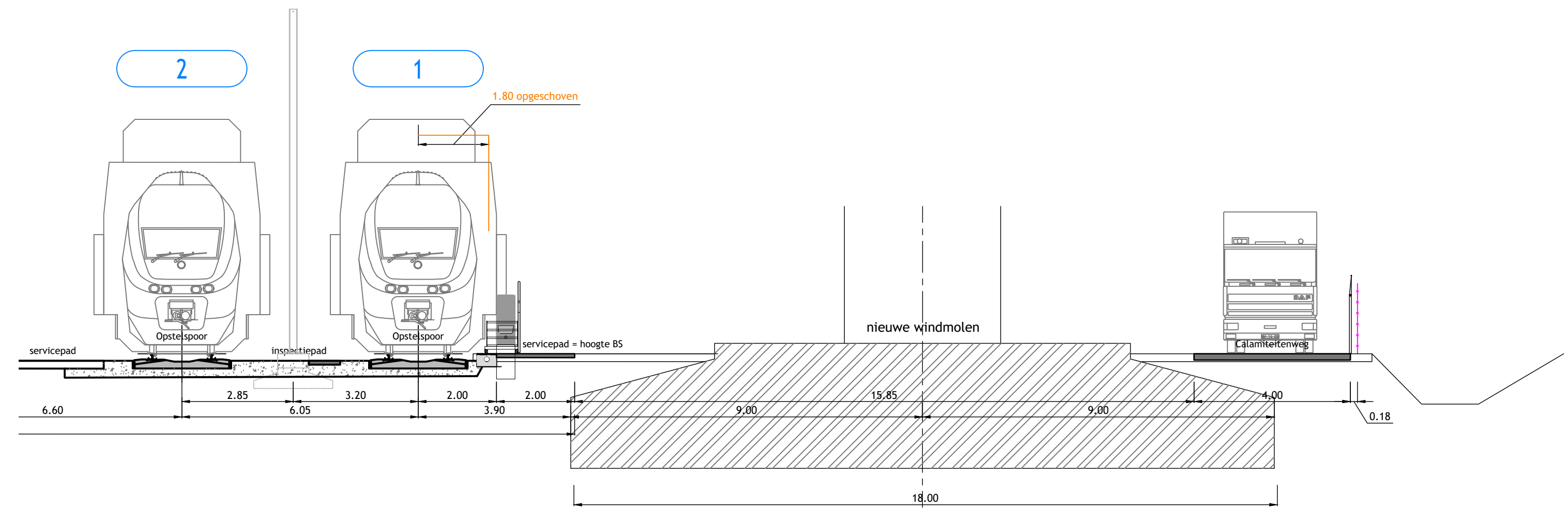
Detail Windmolenspooren schaal 1:100
