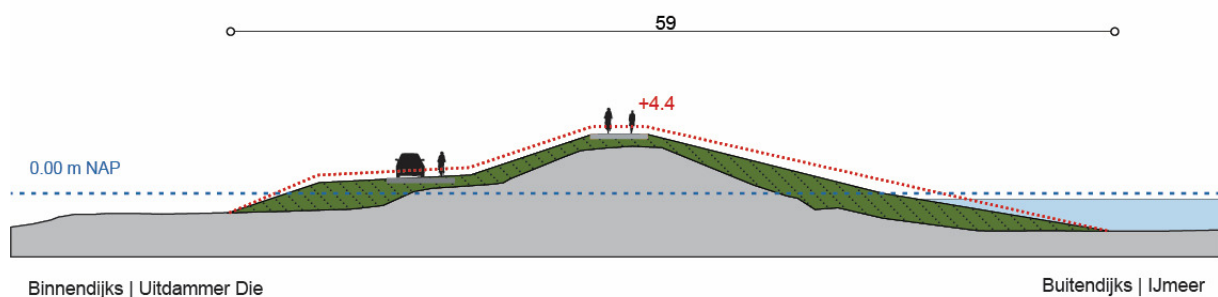
Figuur 93: Maatgevend profiel van de dijk ter hoogte van Uitdammer Die
