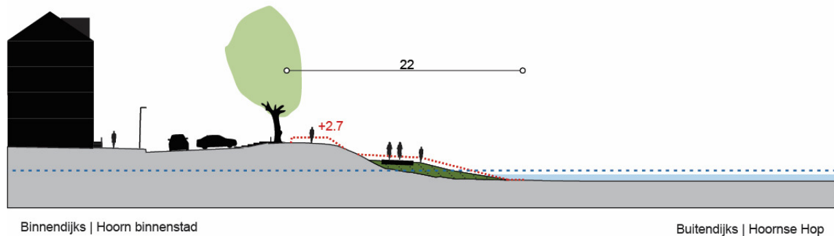
Figuur 42: Matgevend profiel van de dijk ter hoogte van de Hoornse Binnenstad
