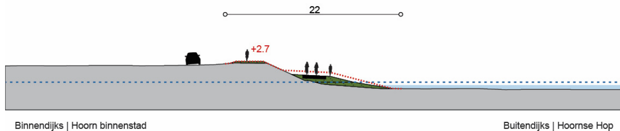
Figuur 43: Matgevend profiel van de Westerdijk (westzijde)
