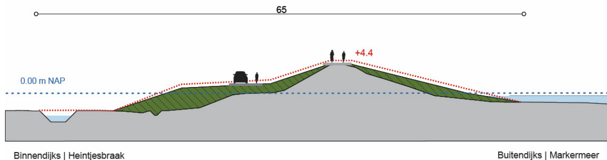
Figuur 64: Maatgevend profiel Heintjesbraak (sectie HE-8-A3 tot en met HE-8-A5)
