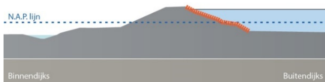
Figuur 27: Veiligheidsprobleem kwaliteit van de bekleding
