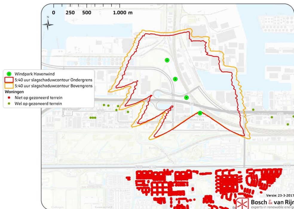
Figuur 3 – 5:40u slagschaduwcontouren van de onder- en bovengrens. Hierbij zijn ook woningen van derden weergegeven. Dit zijn immers de objecten waarvoor de norm geldt. (Er liggen geen andere gevoelige objecten, zoals scholen en ziekenhuizen, binnen of nabij de contour.
