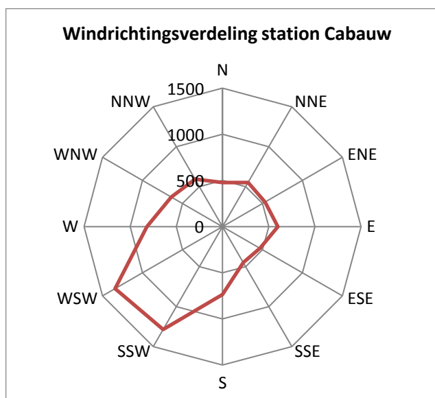
Figuur 2 – Windroos van meteostation Cabauw op 140 meter hoogte.
