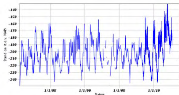
Figuur 60 Peilput B14G0084 filter 001.
