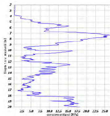
Figuur 38. Sondering ter plaatse van circa km 7.
