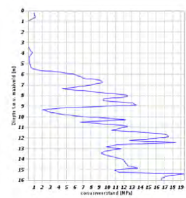
Figuur 24. Sondering ter plaatse van circa km 5.
