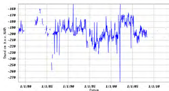
Figuur 49 Peilput B14E0109 filter 001 km 9.
