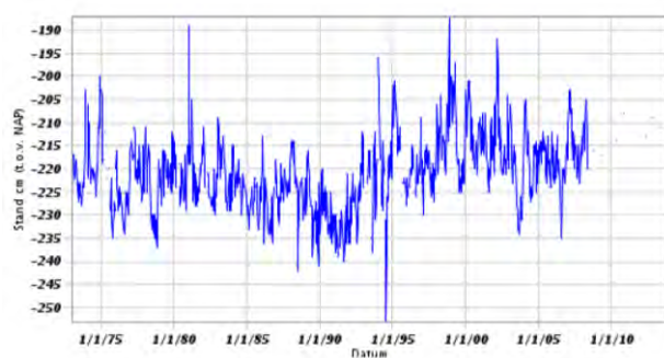
Figuur 81 Peilput B14G0064 filter 001.
