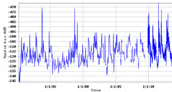
Figuur 53 Peilput B14E0083 filter 001 km 20.
