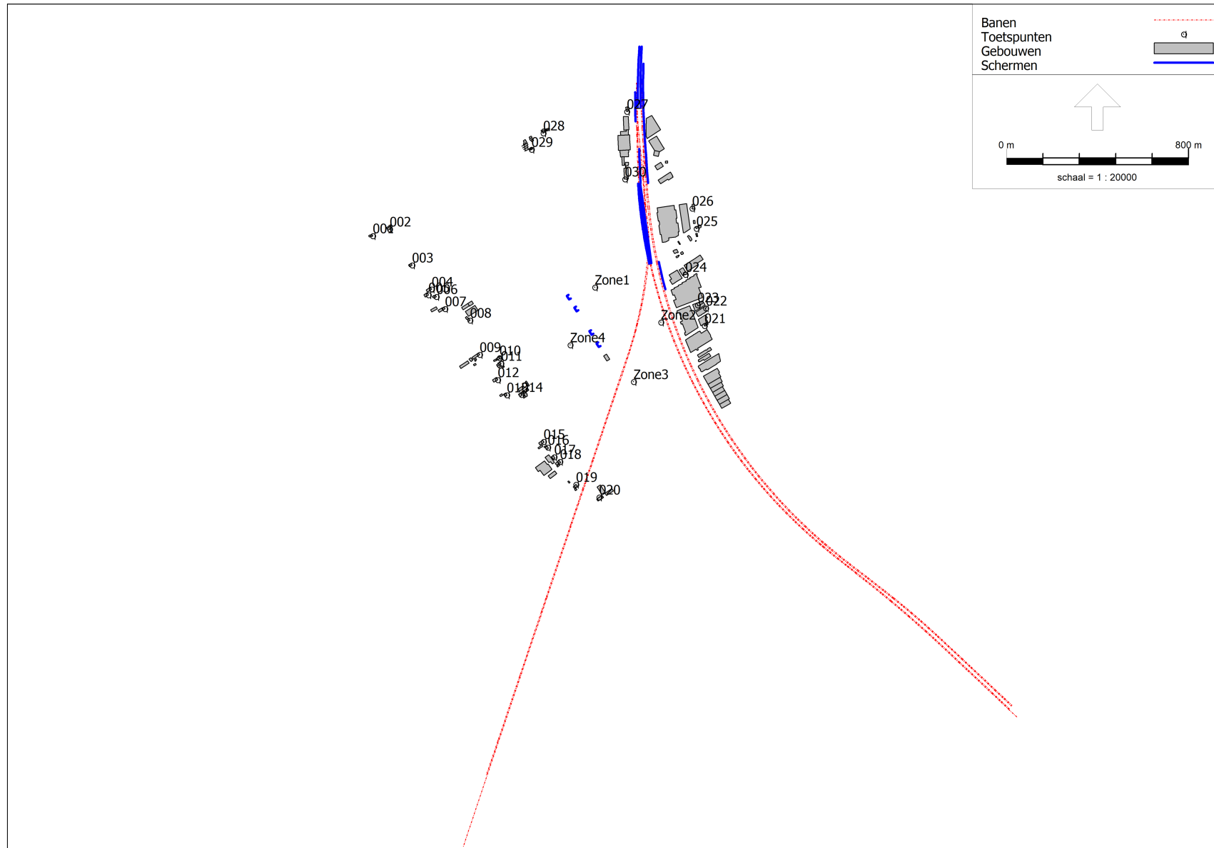
Figuur 1.6 Overzicht rekenmodel railverkeerslawaaï
