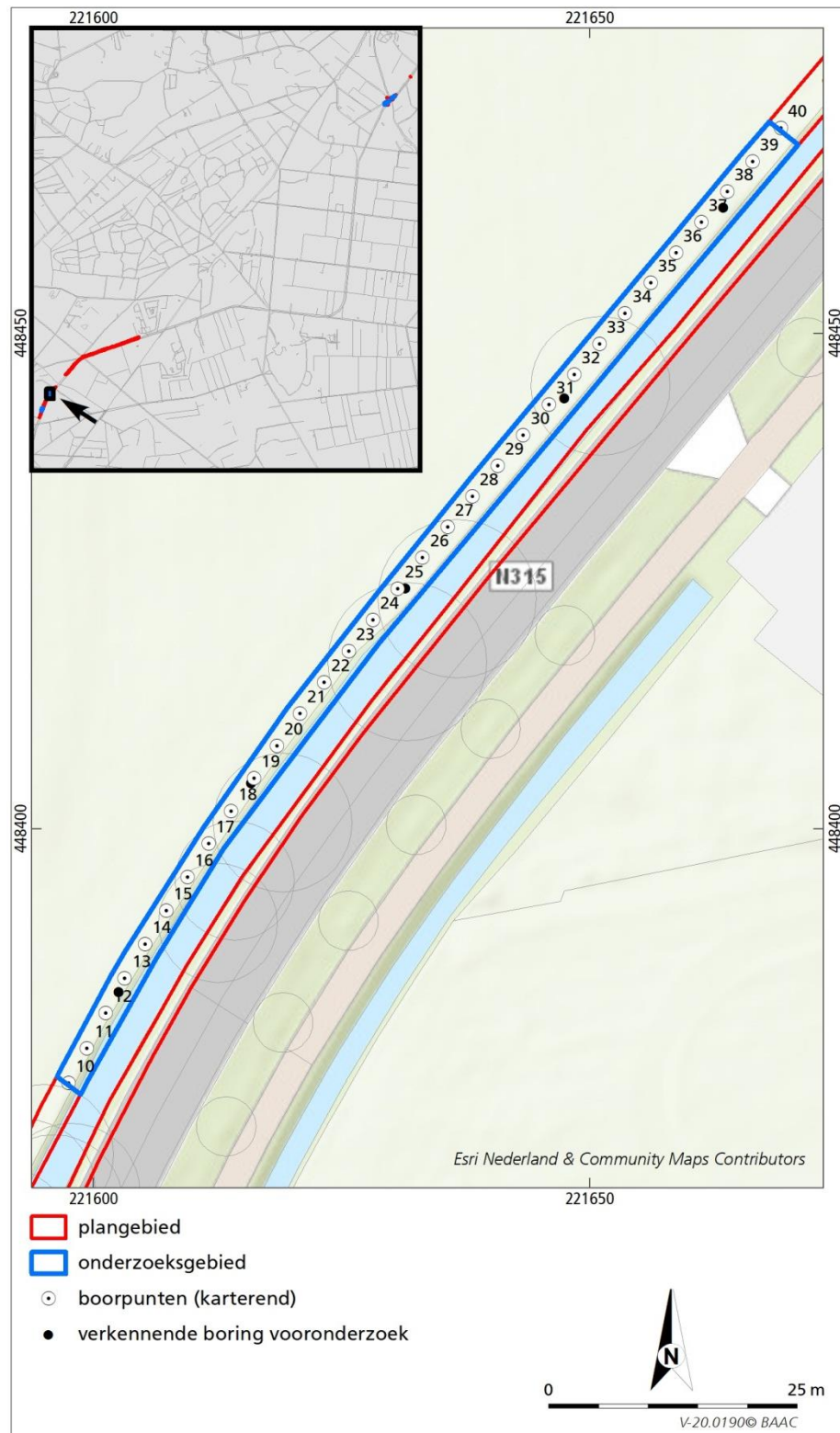
Figuur 2.2 Boorpuntenkaart km 12,75-12,9. Rood omlijnd is de contour van het inventariserend veldonderzoek (verkennende fase, V-20.0015), blauw omlijnd betreft de zone voor onderhavig inventariserend veldonderzoek (karterende fase).
