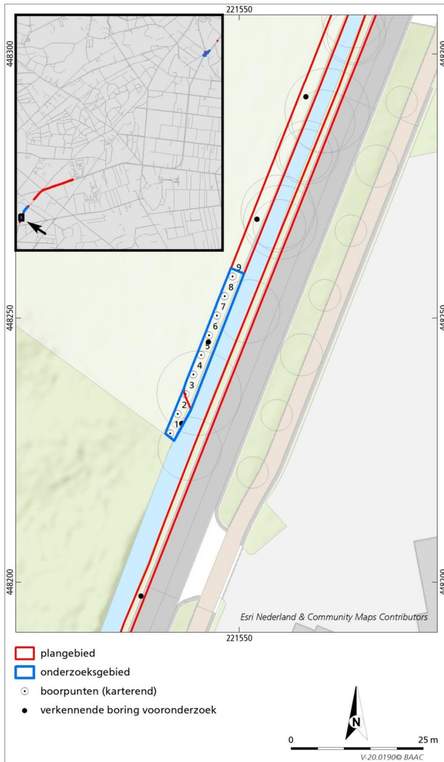
Figuur 2.1 Boorpuntenkaart km 12,65-12,7. Rood omlijnd is de contour van het inventariserend veldonderzoek (verkennende fase, V-20.0015), blauw omlijnd betreft de zone voor onderhavig inventariserend veldonderzoek (karterende fase).
