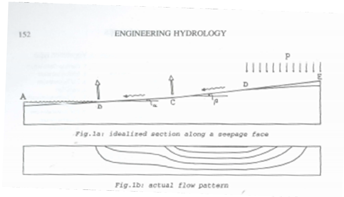
Figuur 38 Schematische voorstelling stromingsprocessen, infiltratie en kwel in een hellend gebied (Maas en Jansen, 1993)
