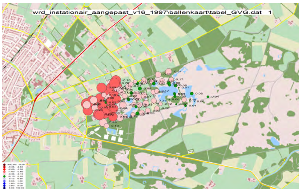
Figuur 3: Validatieresultaat grondwatermodel op basis van grondwaterstandmetingen in peilbuizen 3 maart 2017 door Hullenaar (representatief voor GVG-situatie)
