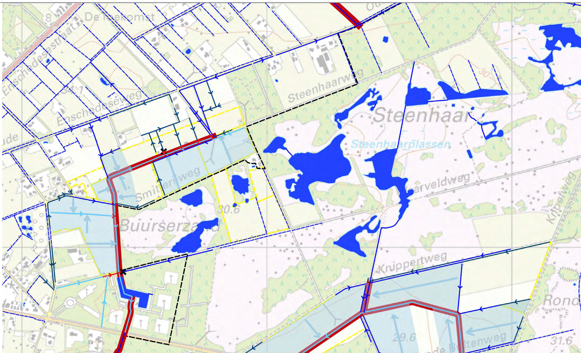
Figuur 3.5: Huidige ontwatering Buurserzand, invloedsgebied BZ1
