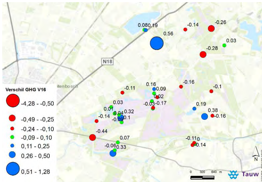
Figuur 1 IJkingsresultaat grondwatermodel Buurserzand, GHG-situatie (bron: Modeloptimalisatie Buurserzand, augustus 2017, Tauw).
