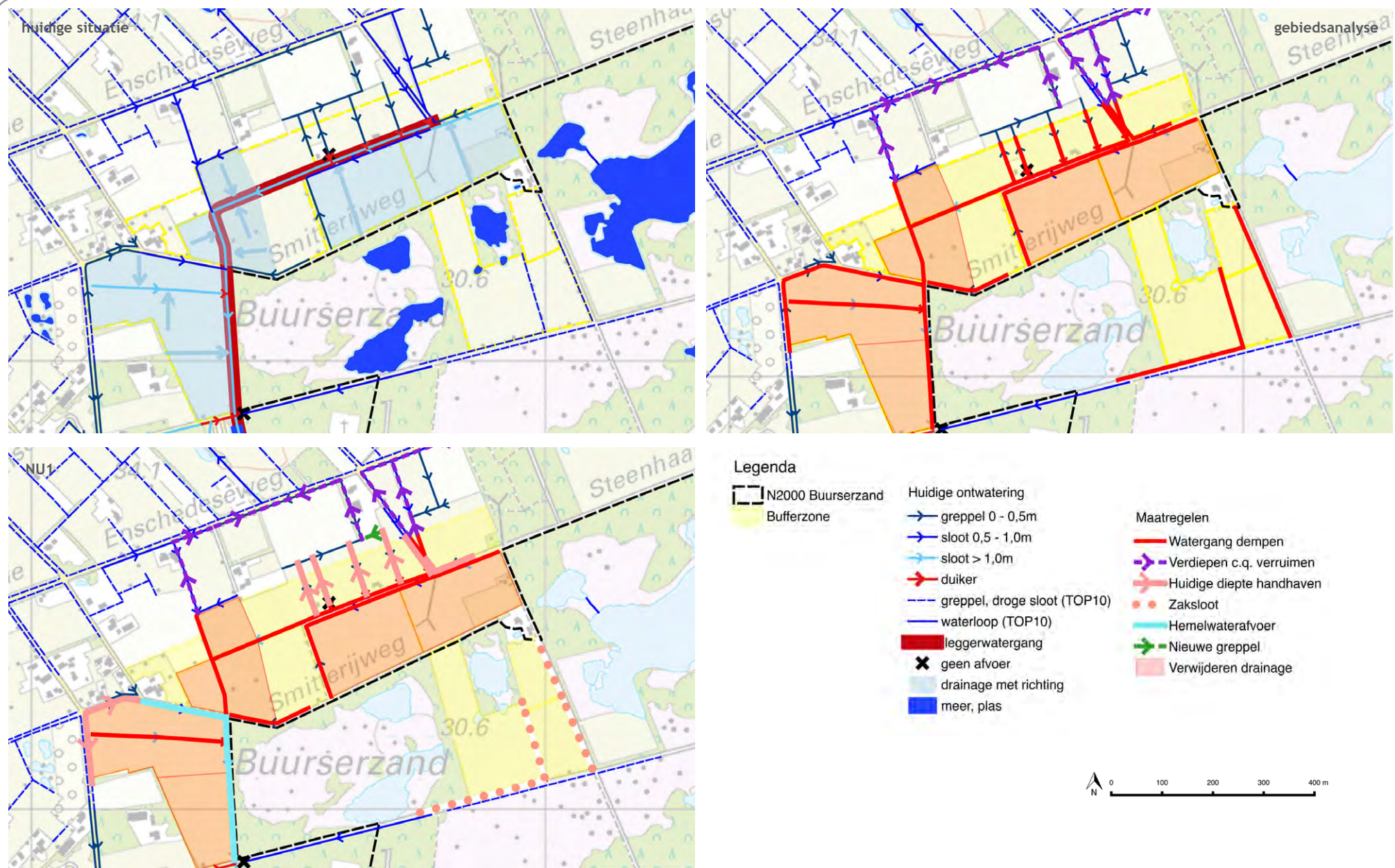
Figuur 4.1: Huidige situatie (linksboven), maatregelen gebiedsanalyse (rechtsboven), maatregelen nadere uitwerking 1 (linksonder)
