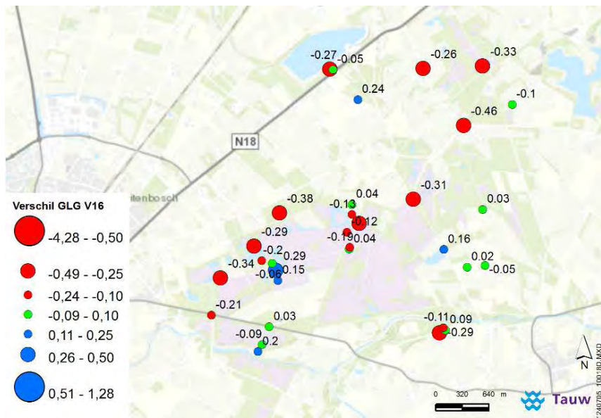
Figuur 2 IJkingsresultaat grondwatermodel Buurserzand, GLG-situatie (bron: Modeloptimalisatie Buurserzand, augustus 2017, Tauw)
