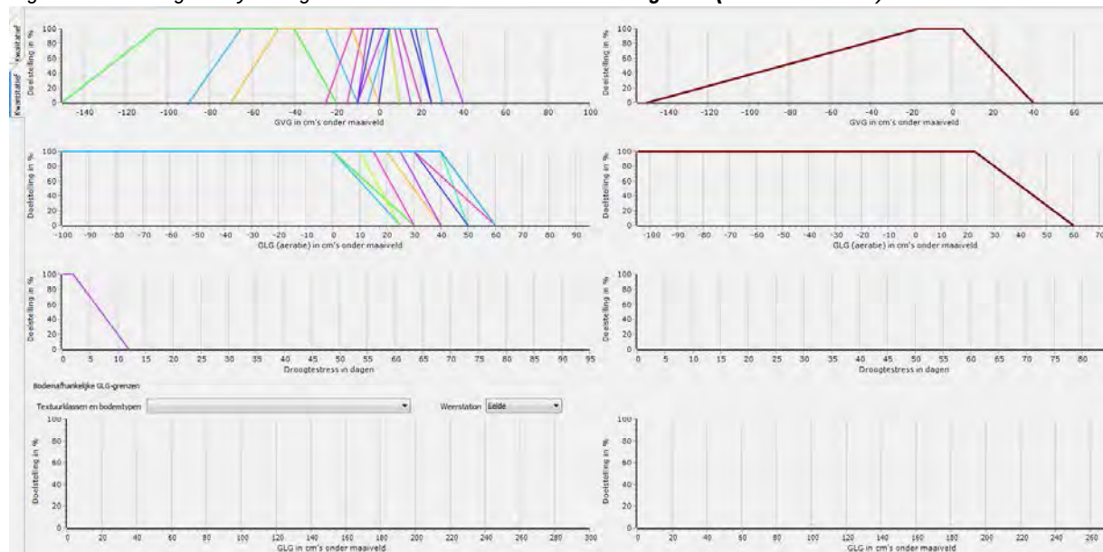
Figuur 3.3. Weergave hydrologische randvoorwaarden Actief hoogveen (uit Waternood3)
