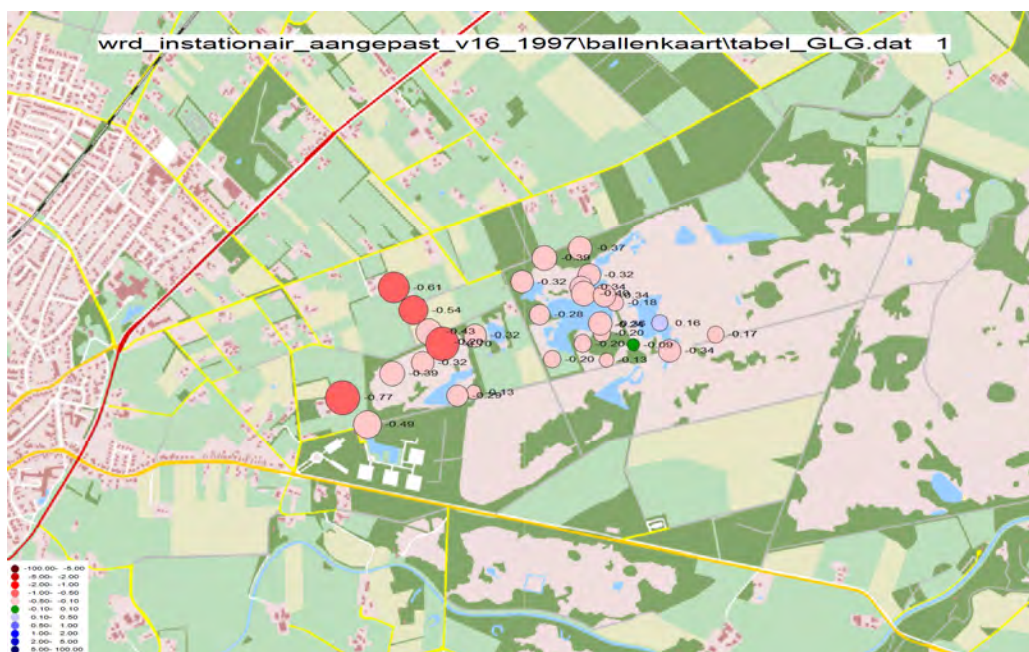
Figuur 4: Validatieresultaat grondwatermodel op basis van grondwaterstandmetingen in peilbuizen 18 juli 2017 door Hullenaar (representatief voor GLG-situatie)
