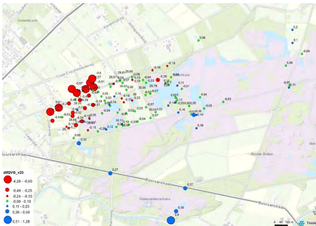
Figuur 6: Resultaat grondwatermodel op basis van grondwaterstandmetingen 3 maart 2017 Hullenaar (representatief voor GVG-situatie)
