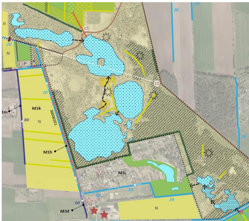
Figuur 4.10 technische uitwerking herstel doorstroomstelsel Bergvennen (legenda zie bijlage 1)
