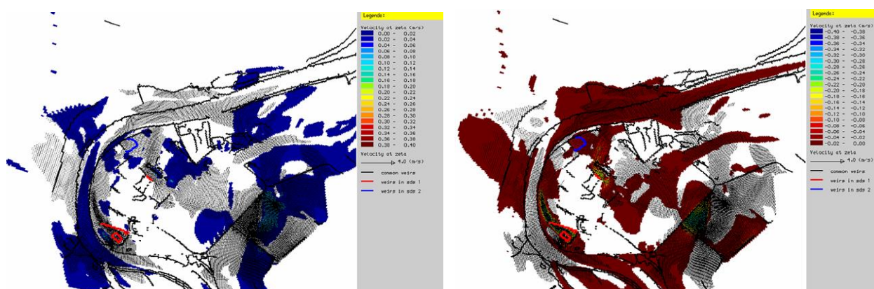
Figuur 5-5: Stroomsnelheidsverschil bij 16.000 m 3 /s - links: sneller stromende gebieden, rechts langzamer stromende gebieden
