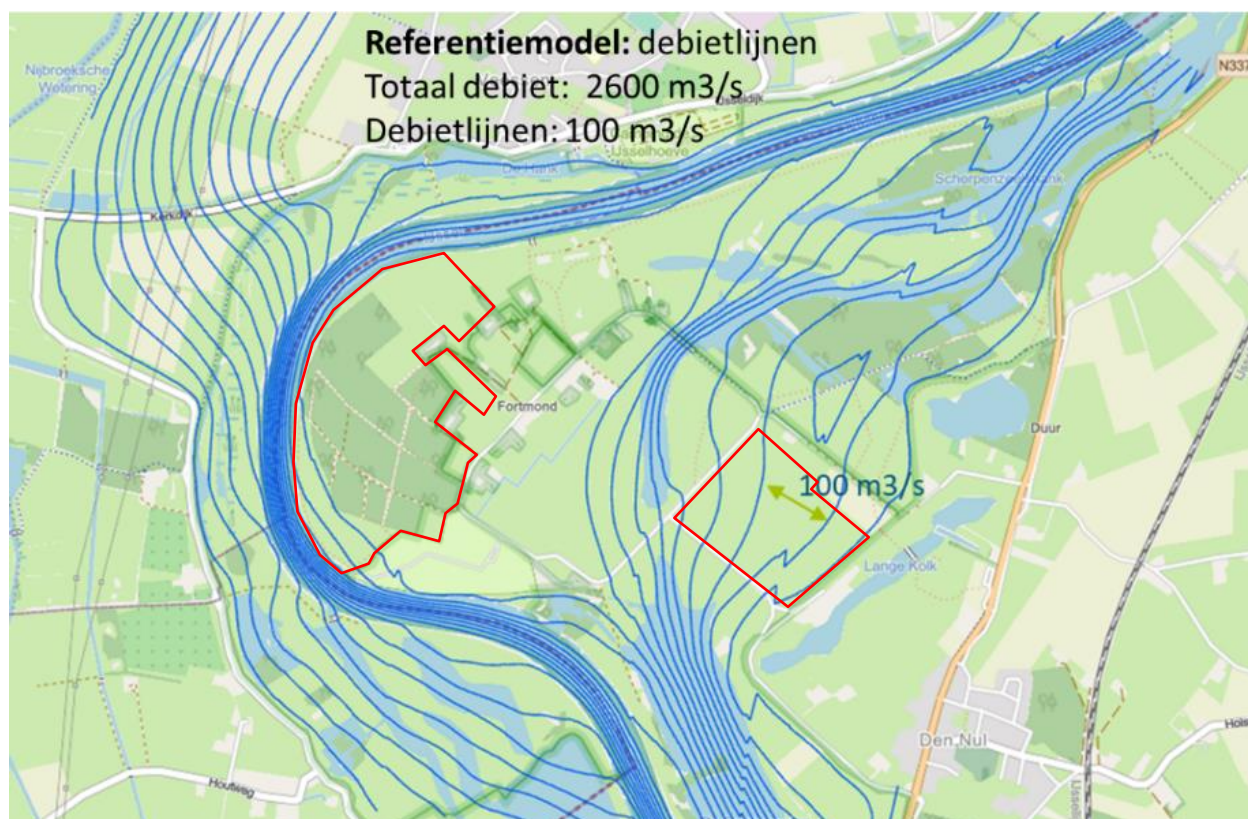
Figuur 2-1 Debietlijnen referentiemodel
