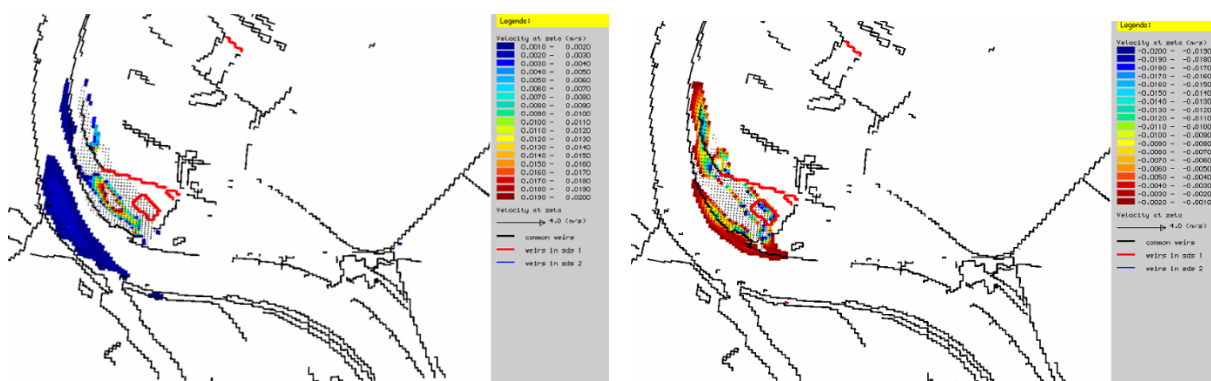
Figuur 5-14: Zoom Achterweerd zuid - Stroomsnelheidsverschil bij 6.000 m 3 /s - links: sneller stromende gebieden, rechts langzamer stromende gebieden
