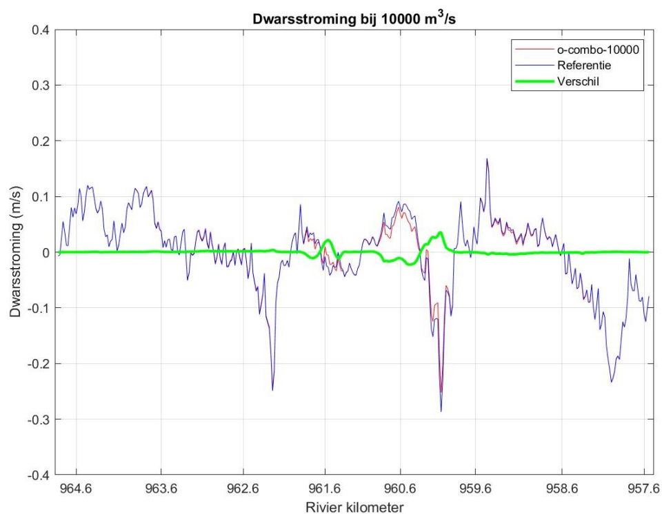
Figuur 5-13: Dwarsstromingsverschil 10.000 m 3 /s op de bakenlijn
