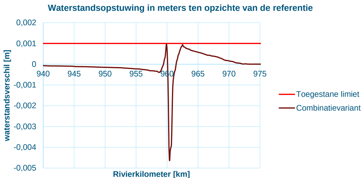
Figuur 5-2: waterstandsverschil op de as van de rivier bij MHW (16.000 m 3 /s) voor de combinatievariant
