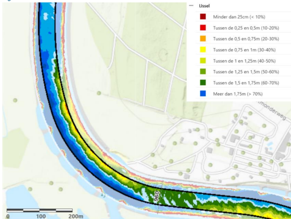
Figuur 5-16: vaardiepte IJssel - bron: waterdieptekaarten RWS, 2024 1
