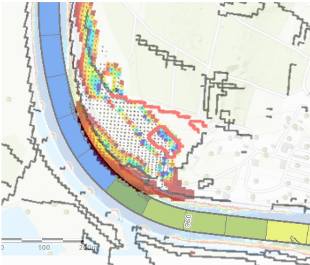
Figuur 5-17: Vaardiepte kaart inclusief stroomvertragende locaties bij 6.000 m 3 /s
