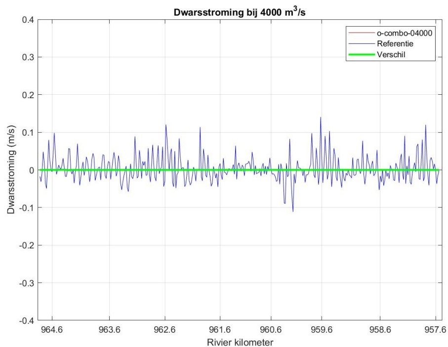
Figuur 5-10: dwarsstromingsverschil 4.000 m 3 /s op de bakenlijn
