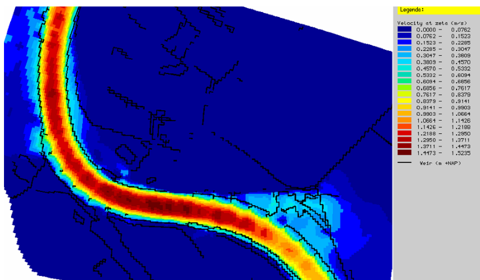
Figuur 5-15: Stroomsnelheid referentie 6.000 m3/s
