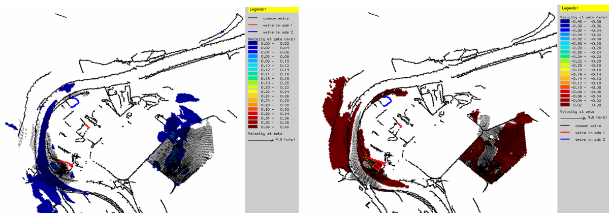
Figuur 5-8 Stroomsnelheidsverschil bij 8.000 m³/s - links: sneller stromende gebieden, rechts langzamer stromende gebieden
