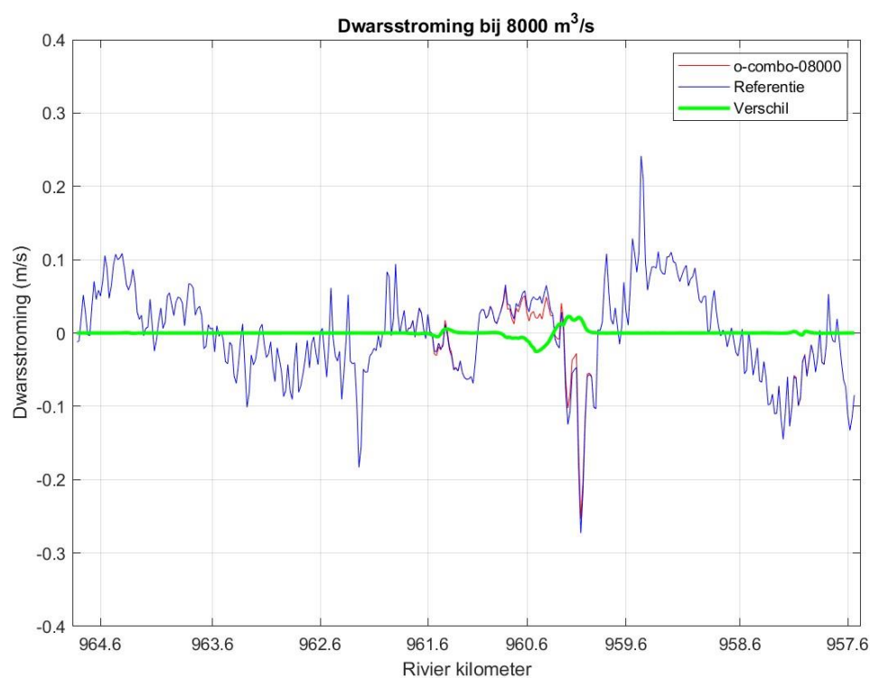
Figuur 5-12: Dwarsstromingsverschil 8.000 m 3 /s op de bakenlijn
