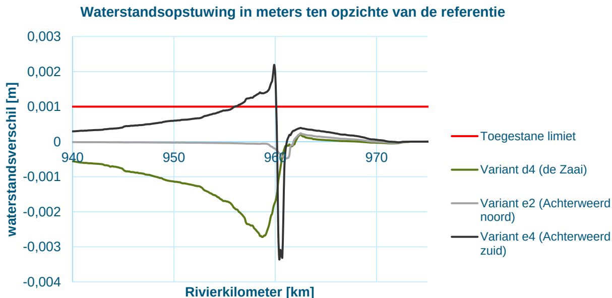
Figuur 5-1: waterstandverschil op de as van de rivier bij MHW (16.000 m 3 /s) voor de drie losse varianten
