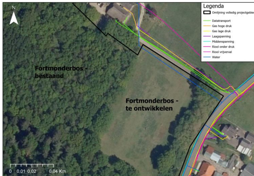
Figuur 4: Ligging van de waterleiding (perceel in eigendom Staatsbosbeheer)
