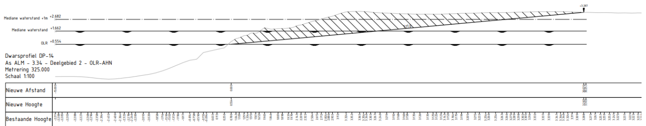
Figuur 5-13 Impressie KRW-inrichting flauwe oeveren ter hoogte van Achterweerd Noord met dwarsprofiel
