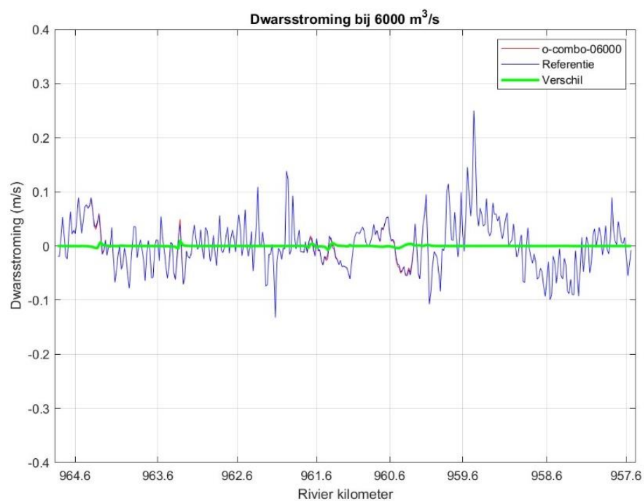
Figuur 5-11: Dwarsstromingsverschil 6.000 m 3 /s op de bakenlijn
