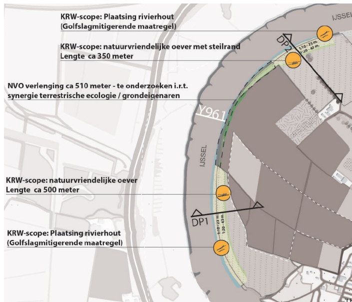
Figuur 3-15: Schetsontwerp beoogde KRW maatregelen (bovenaanzicht) als vertrekpunt voor inrichting van de oevers ter hoogte van Achterweerd Noord en Achterweerd Zuid (bron: GROW).
