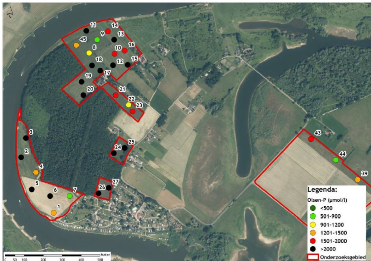
Figuur 3-4 Gemeten Olsen-P concentraties van de bovengrond (0-15 cm -mv) (B-Ware, 2023)
