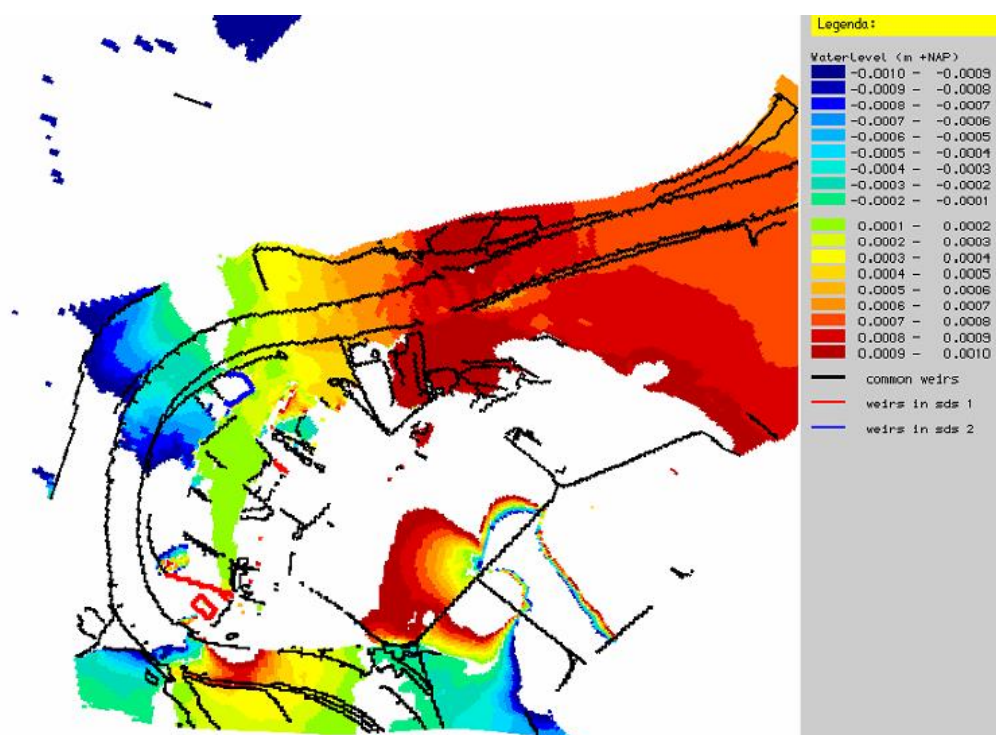
Figuur 5-4: Effecten onder de 1 mm (opstuwing geel-rood en waterstandsvaling blauw-groen)
