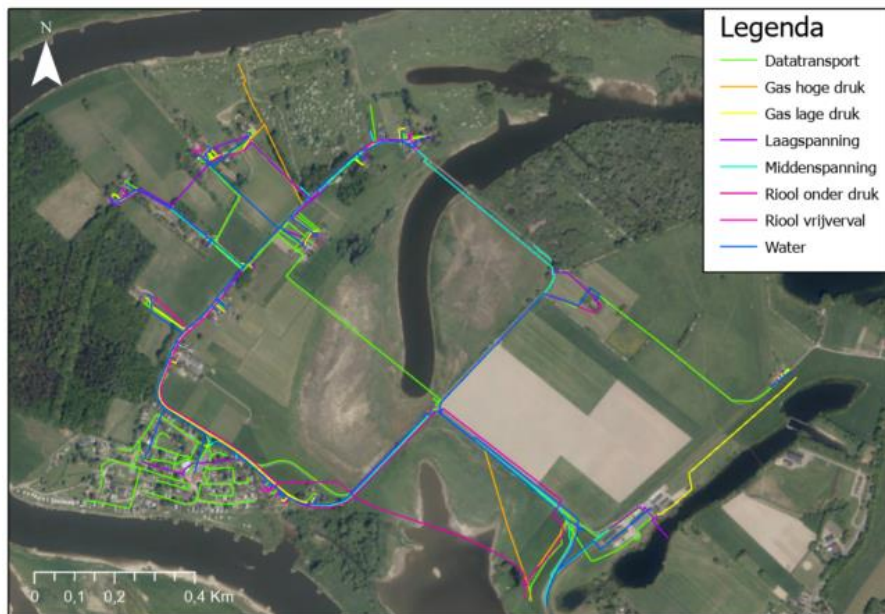
Figuur 2: overzicht alle kabels en leidingen in en om het projectgebied.
