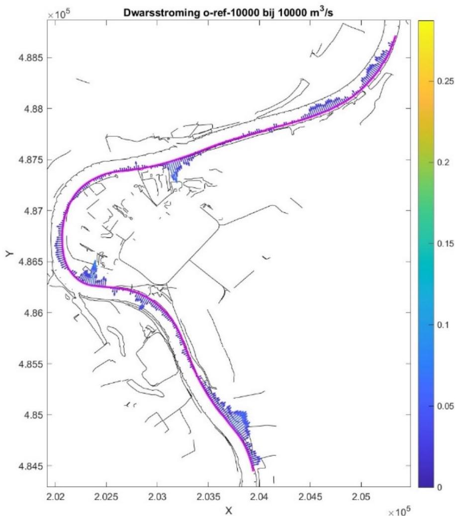
Figuur 5-9: Evaluatie dwarsstroming referentie 10.000 m 3 /s
