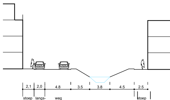
Doorsnede gebiedsontsluitingsweg, deelgebied A (2)
