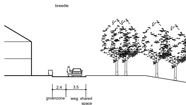
Doorsnede deelgebied C1
