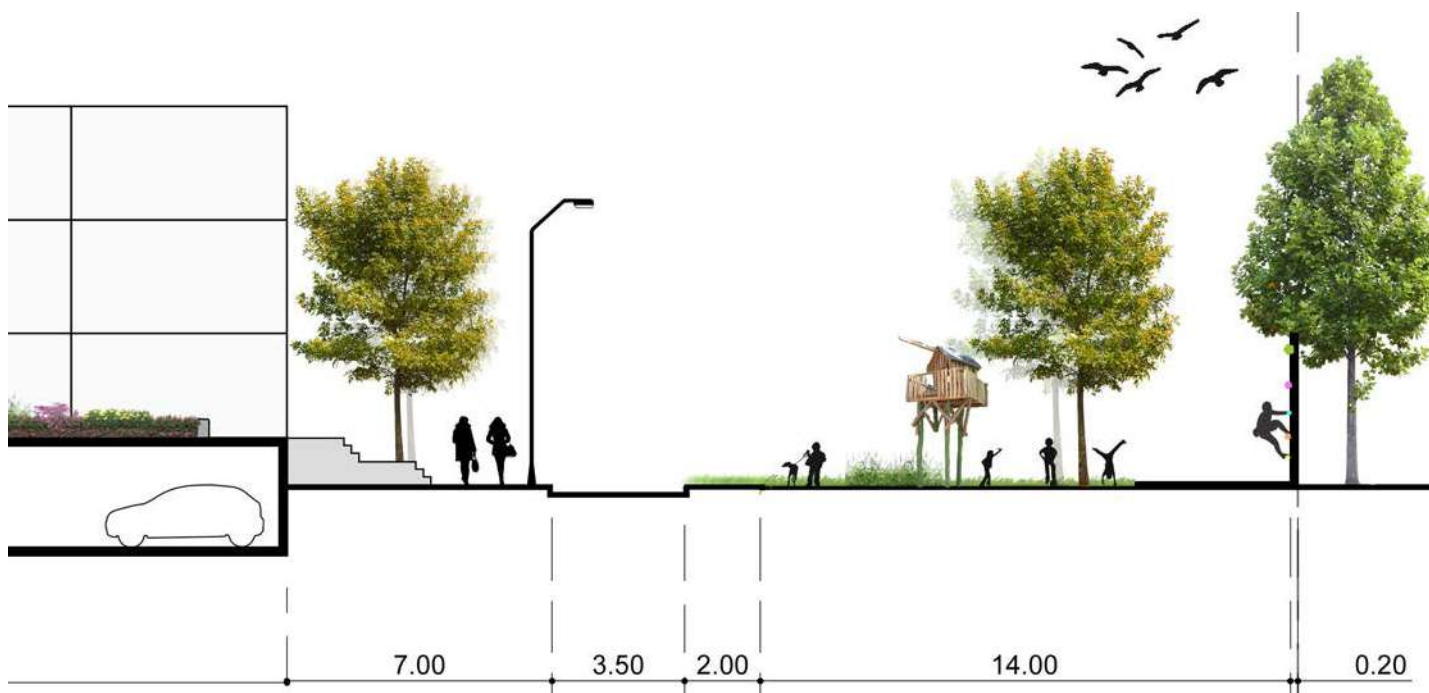
Doorsnede over plantsoen en geluidsmuur ter plaatse van klimmuur/ speelplek
