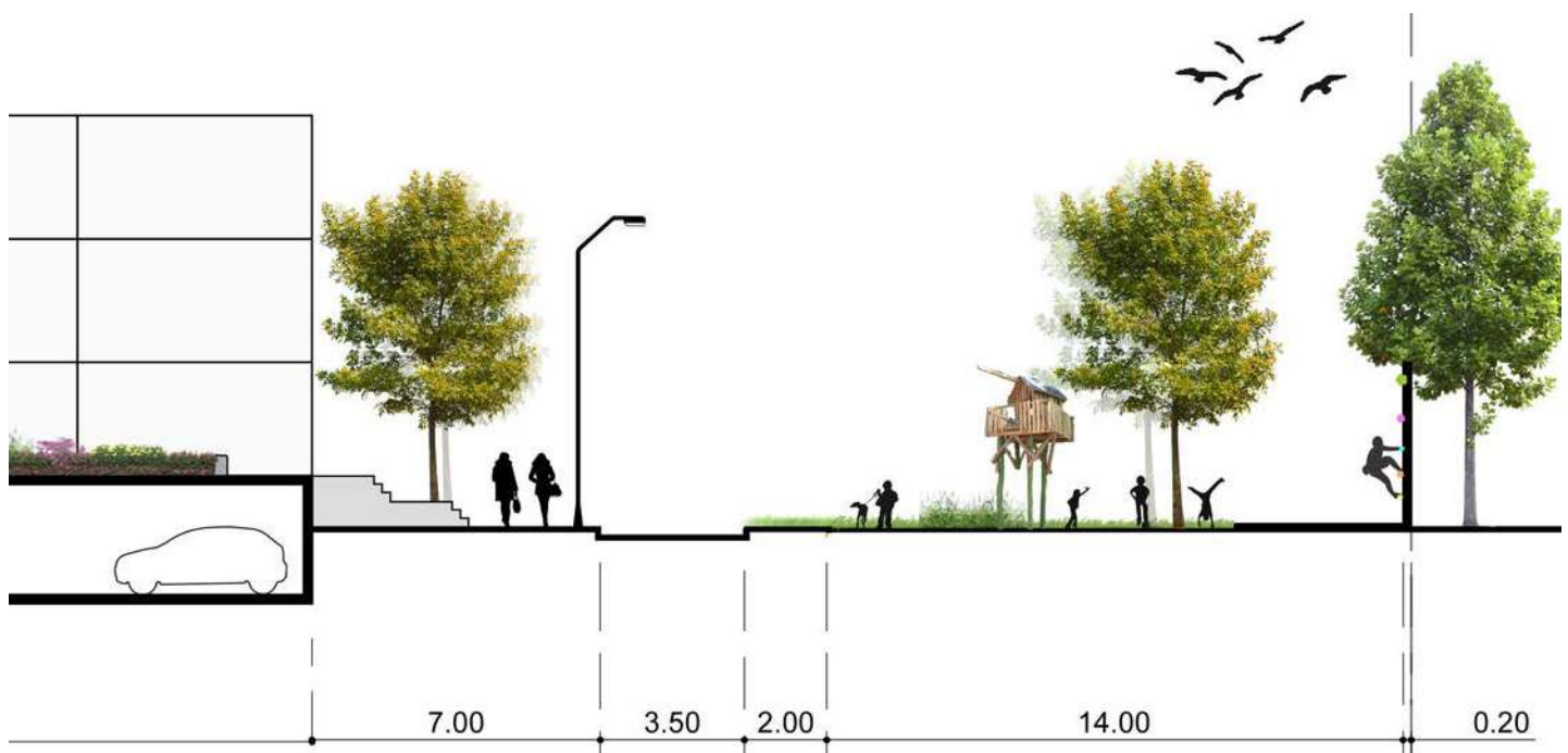
Doorsnede over plantsoen en geluidsmuur ter plaatse van klimmuur/ speelplek
