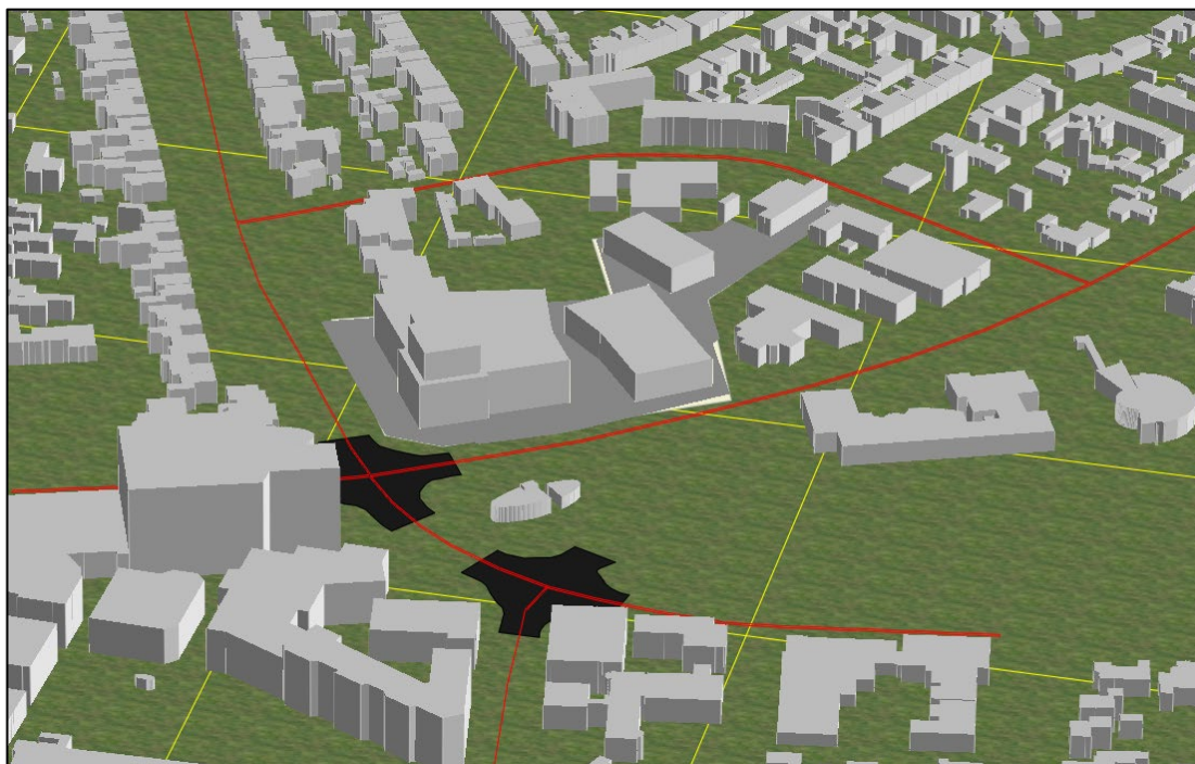
Figuur 4.1: Akoestisch rekenmodel, 3D weergave
