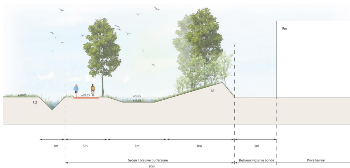
Doorsnede westelijke groenzone
