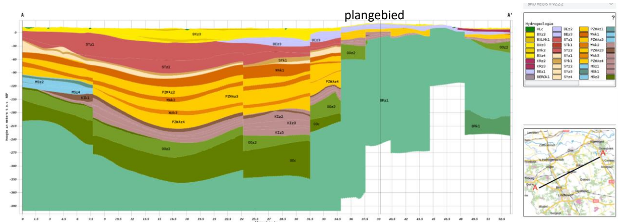
Figuur 2-8: Dwarsdoorsnede van het ondergrondmodel REGIS voor zuidoost Brabant, met ter hoogte van de verticale grijze streep het plangebied (bron: DINOloket). De verschillende kleuren zijn afzettingen van verschillende periodes/oorsprong, waarbij in de ondergrond duidelijk sprongen te zien zijn waar breuken voorkomen.
