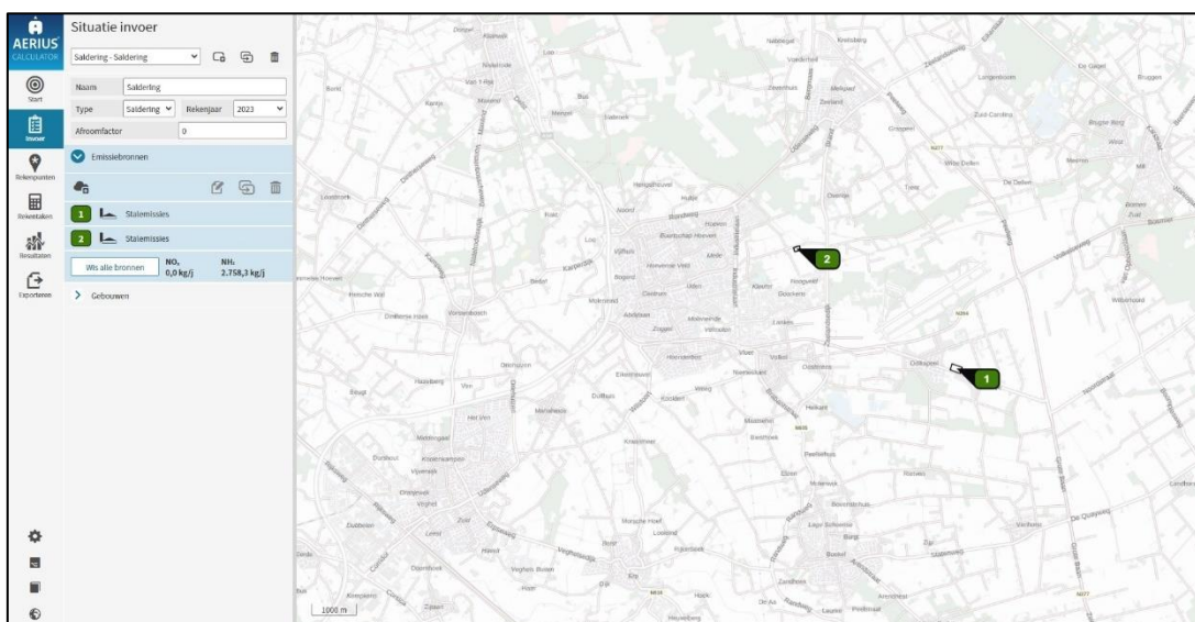
Afbeelding 3 - AERIUS-model referentiesituatie
