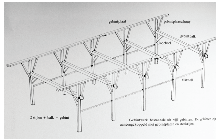
Schematische opbouw van houtskelet van hallenhuis met koppelbalken tussen de gebintstijlen, hier 'steekrij' genoemd.
