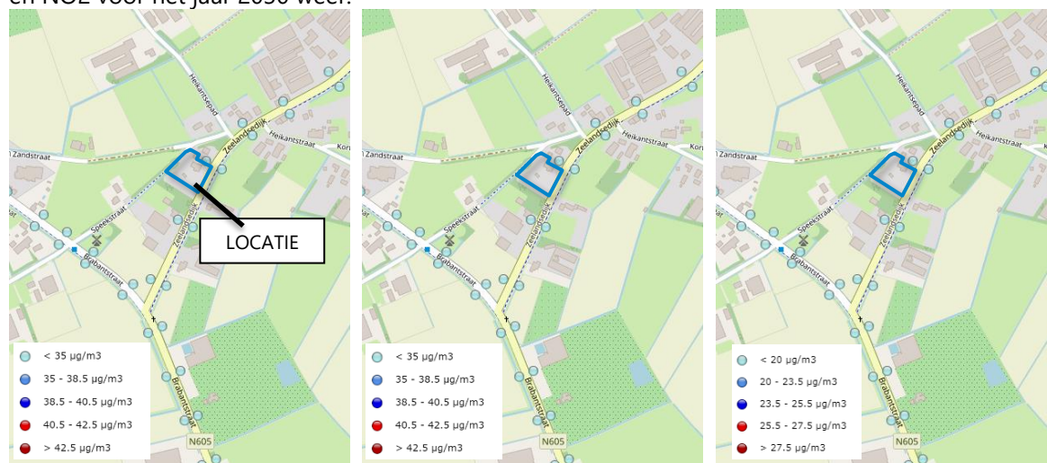
Afbeelding 3 : concentraties NO2 (links), PM10 (midden) en PM2.5 (rechts) voor het jaar 2030
