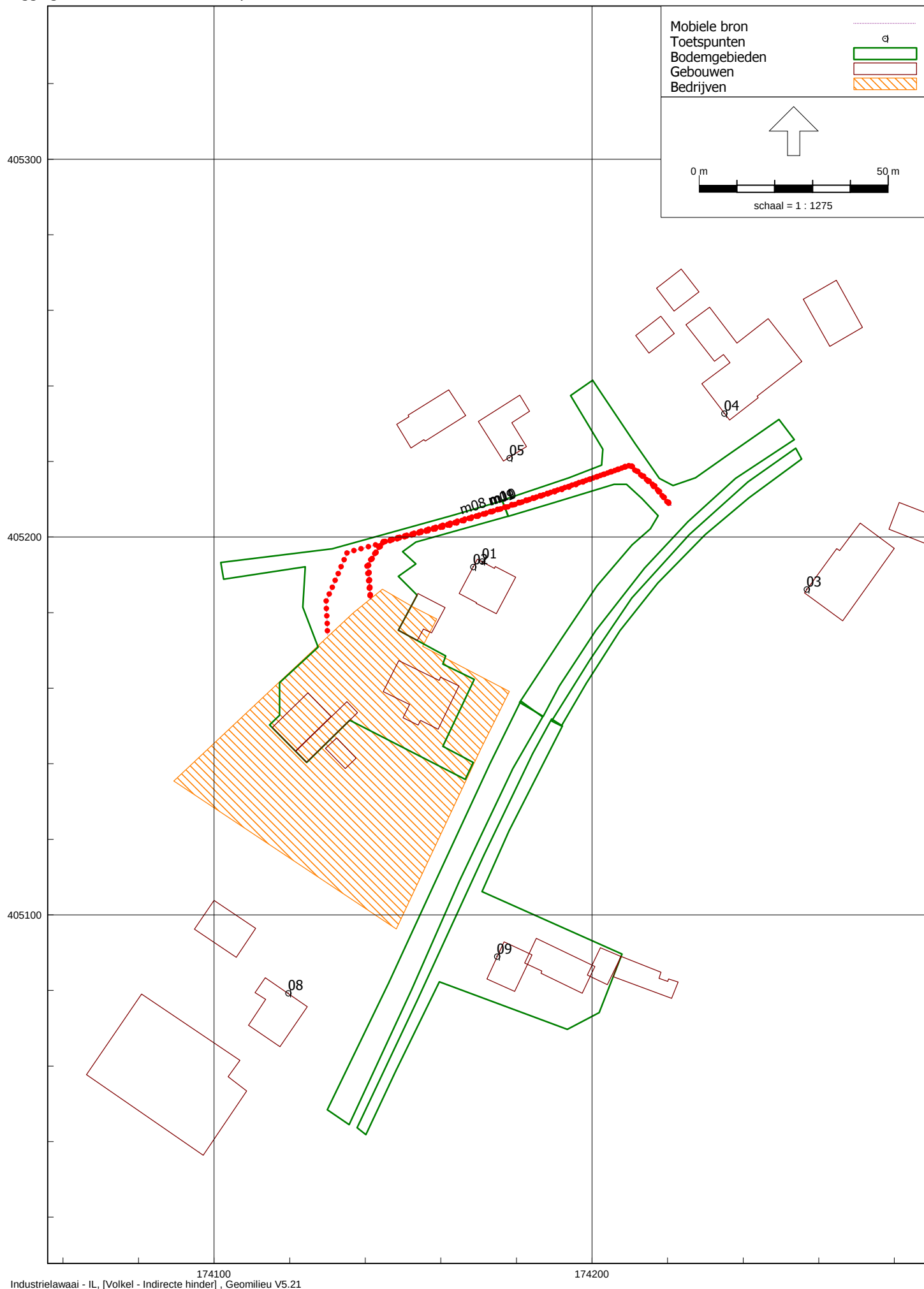
Figuur 9 Ligging mobiele bronnen en rekenpunten indirecte hinder
