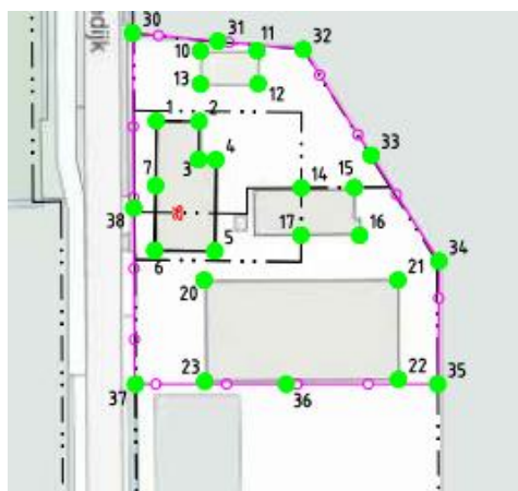
Afbeelding 3: positionering meetpunten
