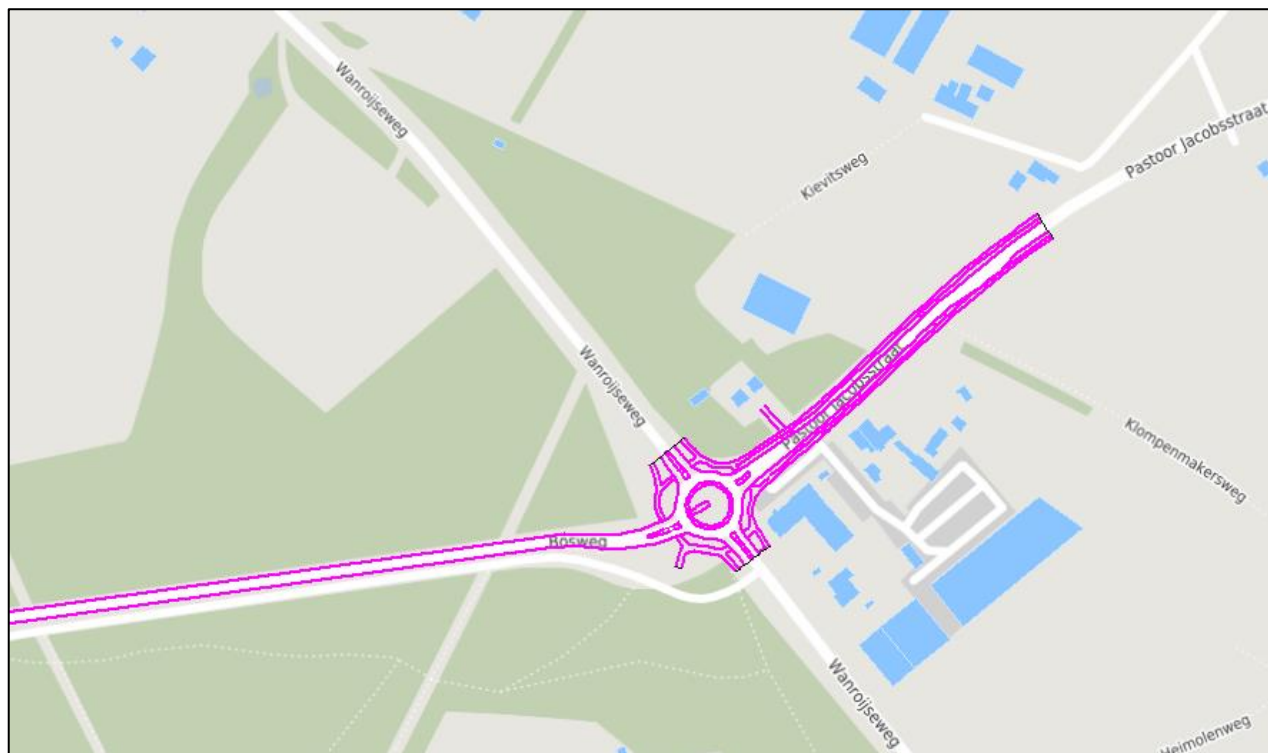
Figuur 4.2c: De ontwerpwijzigingen N264 in deelgebied 3a.
