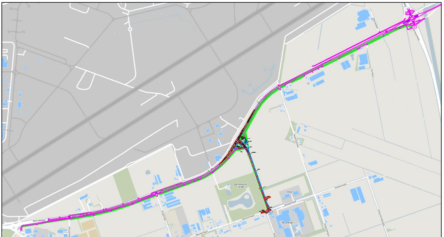
Figuur 4.2a: De ontwerpwijzigingen N264 in deelgebied 1.
