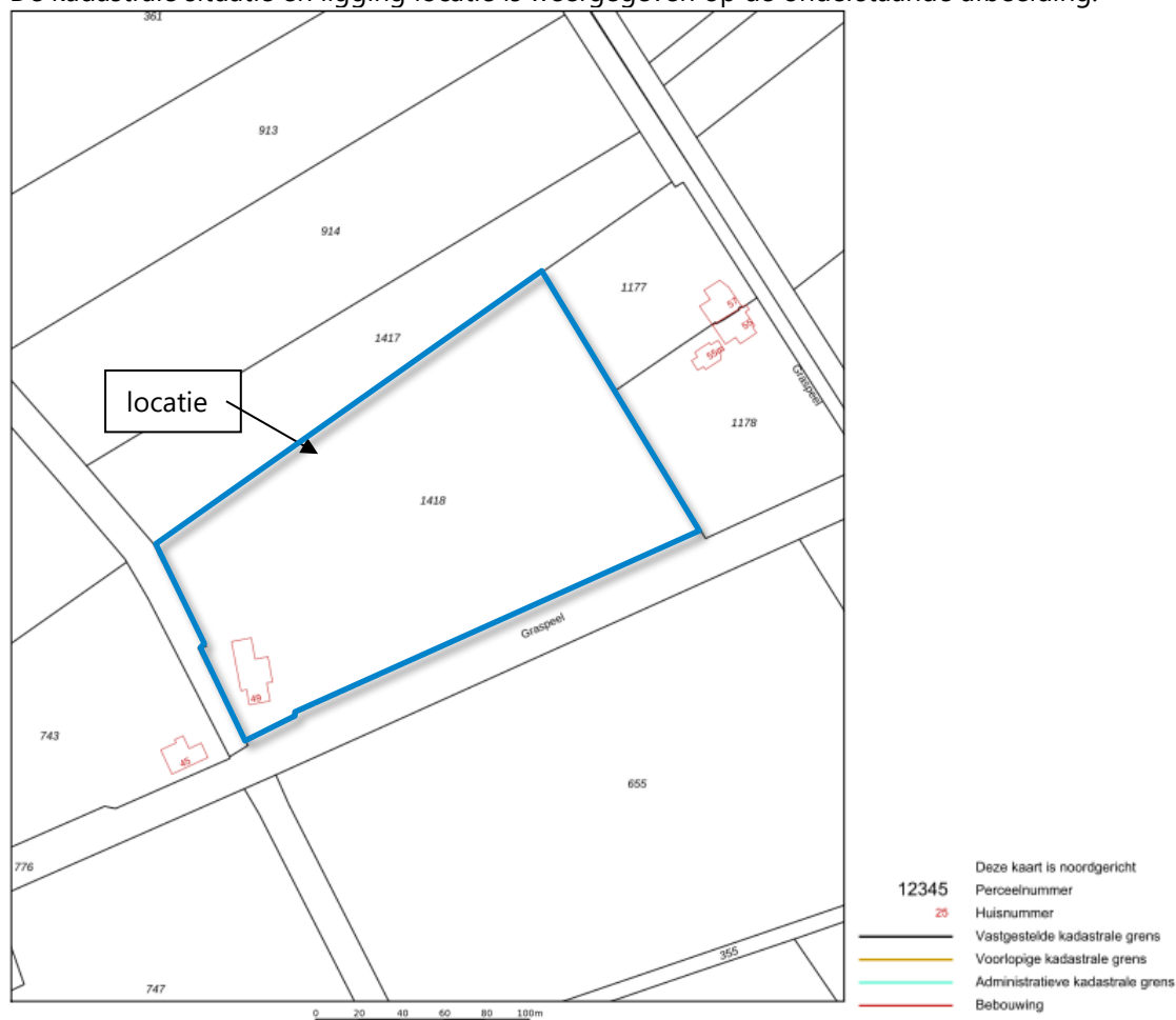
Afbeelding 1: kadastrale kaart
