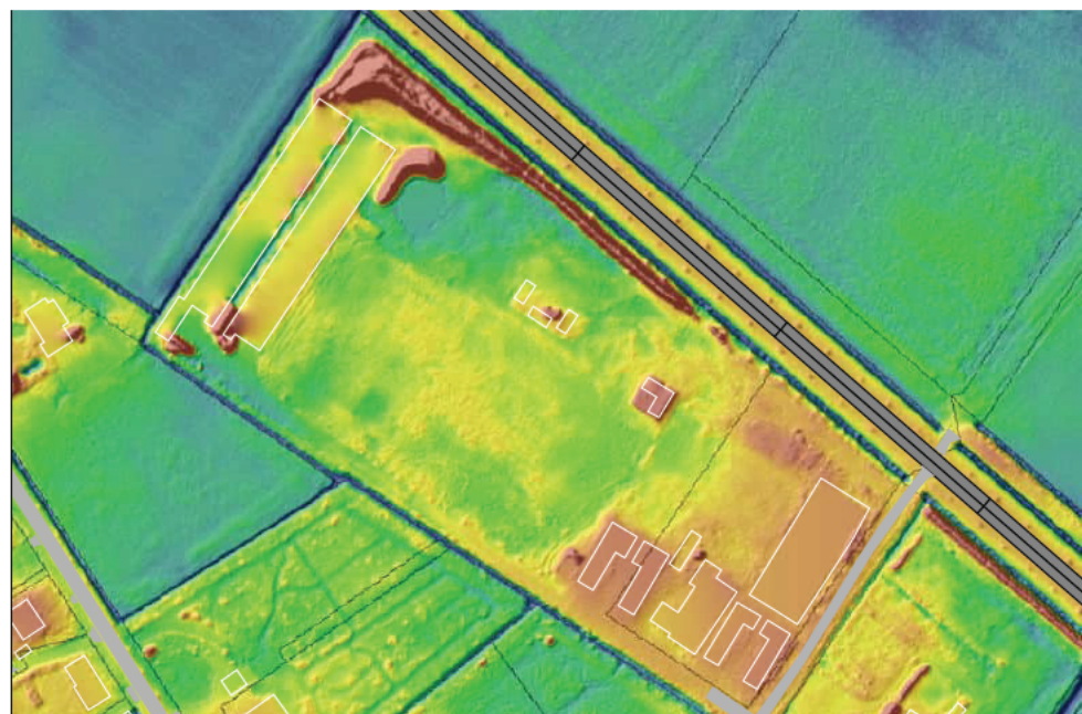
Hoogtekaart (rood is hoog, blauw is laag)
