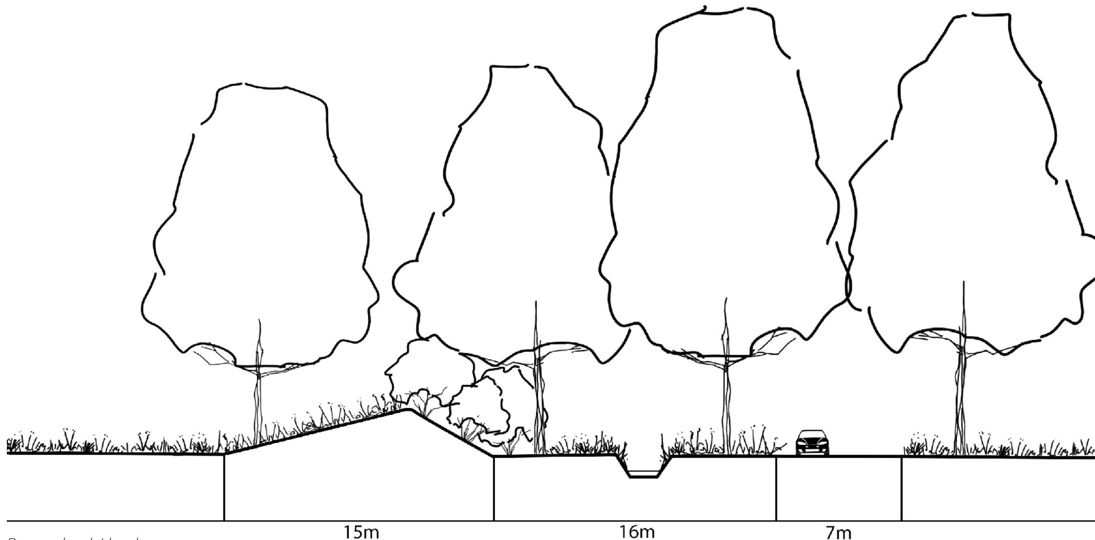
Doorsnede geluidswal
