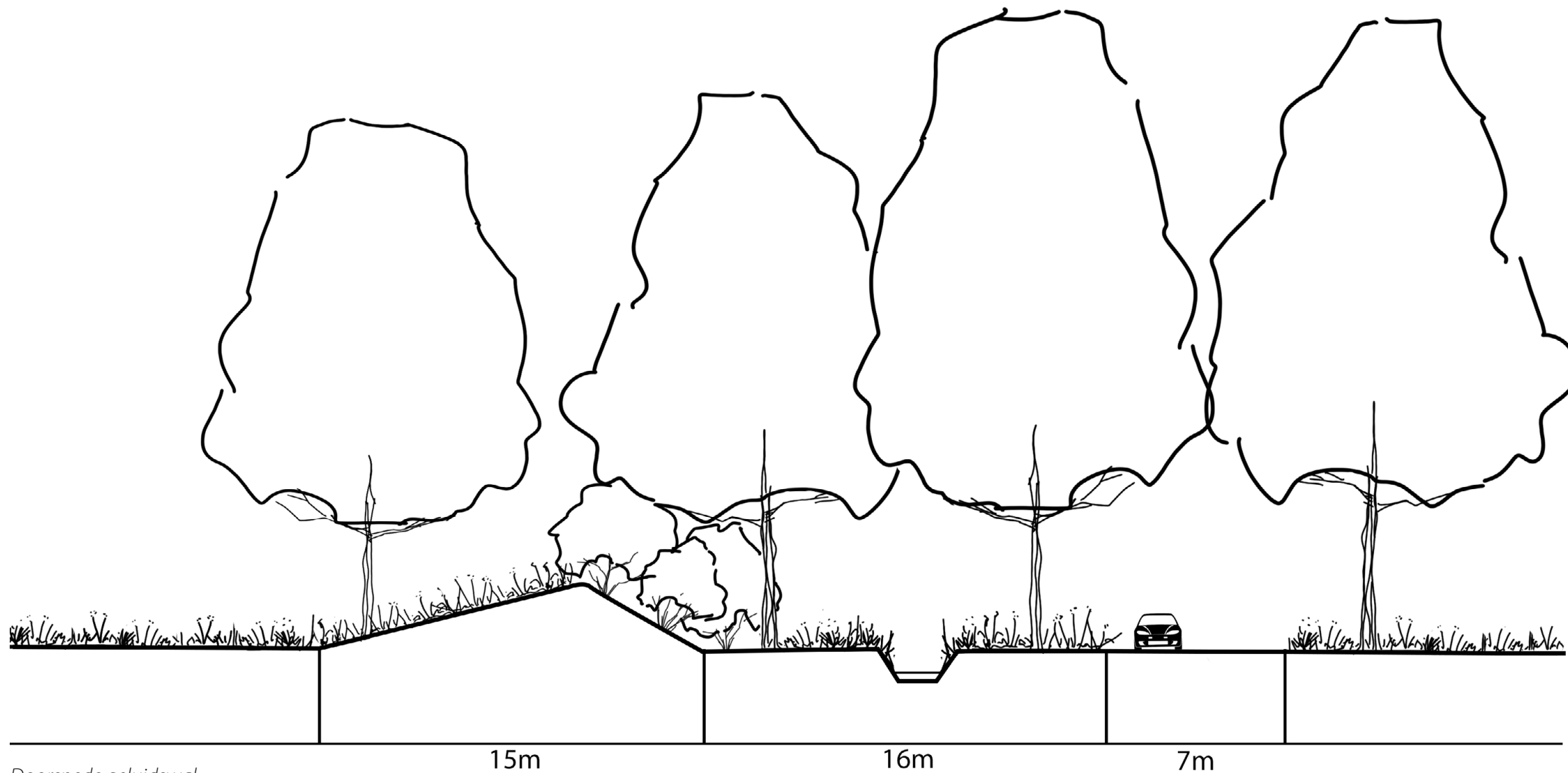
Doorsnede geluidswal
