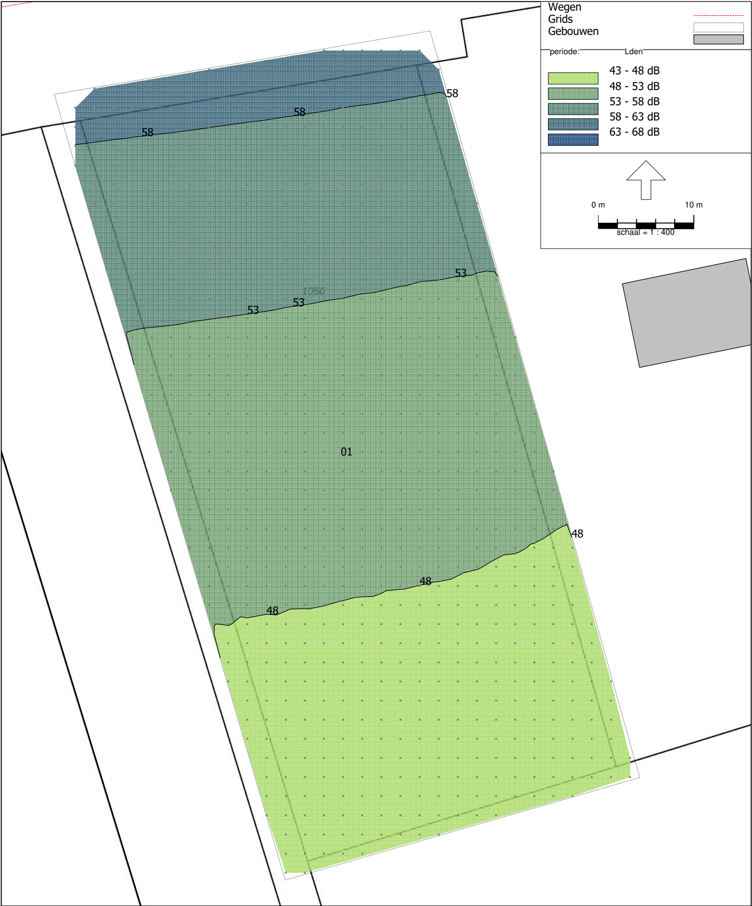
Figuur 3.2 Geluidcontouren 4,5
