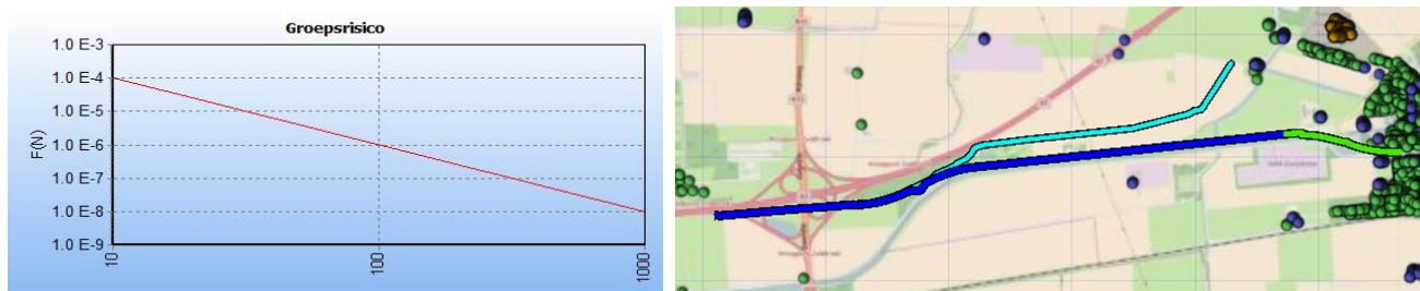
Figuur 6 Links de FN-curve van de kilometer met de hoogste overschrijdingsfactor van tracé 3 van gastransportleiding N-508-50 in de huidige situatie. De ligging van deze kilometer is daarnaast in het groen weergegeven op een topografische kaart.
