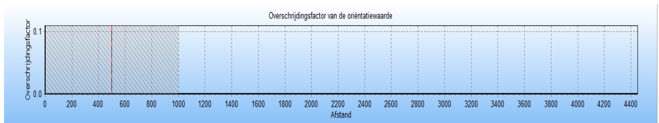
Figuur 7 Overschrijding van het groepsrisico als functie van de stationing van tracé 3 van N-508-50.
