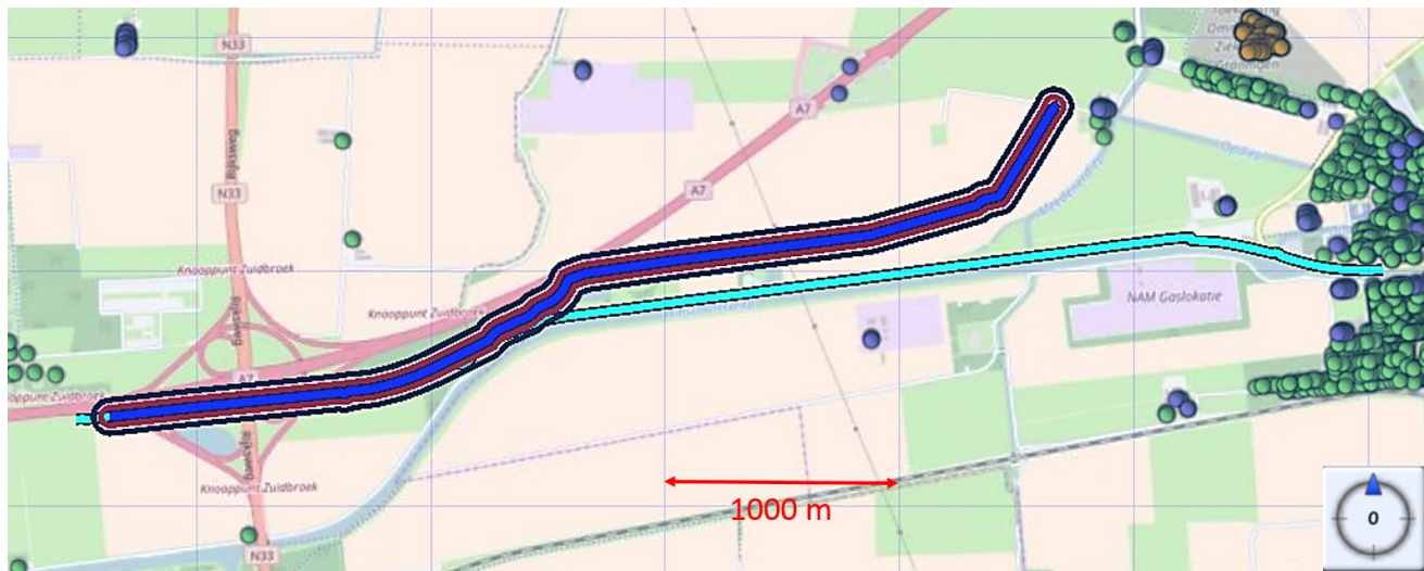
Figuur 2 Bevolkingsgegevens rondom tracé 3 van N-508-50 (toekomstige situatie) zoals aangeleverd door de populateservice van IPO. Groen gekleurde adressen zijn woningen, blauw gekleurde adressen zijn werklocaties en bruin gekleurde adressen zijn evenementen. De zwarte lijn geeft het invloedsgebied (1% letaliteitsgrens) van de leiding weer; het rode gebied geeft de 100% letaliteitsgrens weer.
