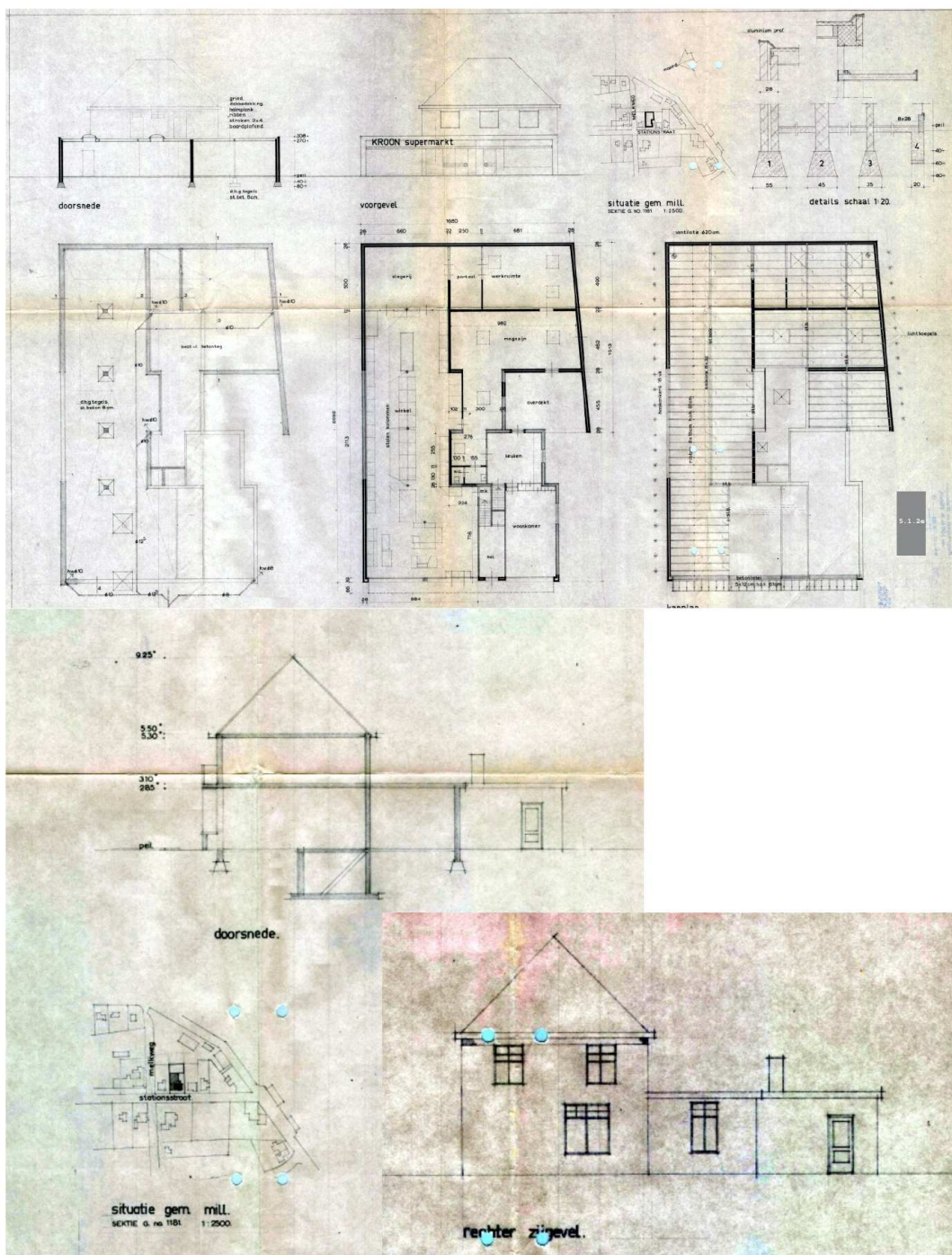
Figuur 10: Bouwtekening uitbreiding van winkelgebouw (boven) en woonhuis (beneden) uit 1968 (Brabants Historisch Informatie Centrum (BHIC) 2022).
