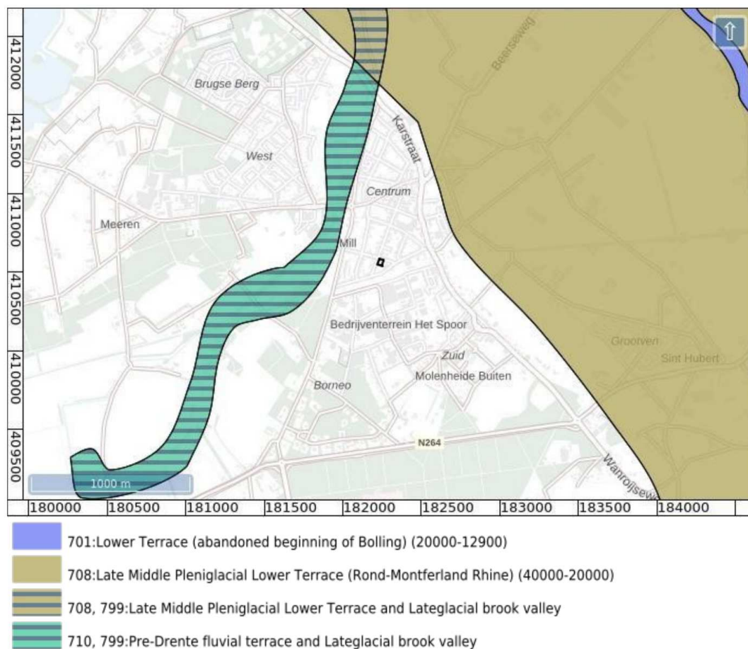
Figuur 12: Beddinggordels Laat Glaciaal - Vroeg Holoceen (Cohen e.a. 2012).
