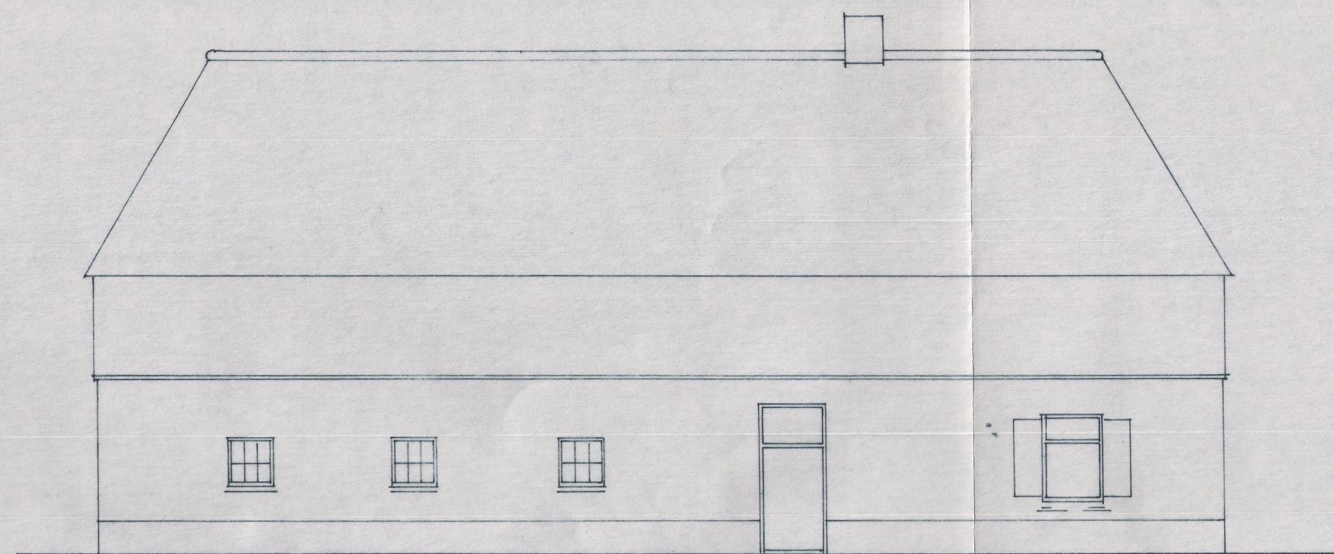
- VOORGEVEL -
