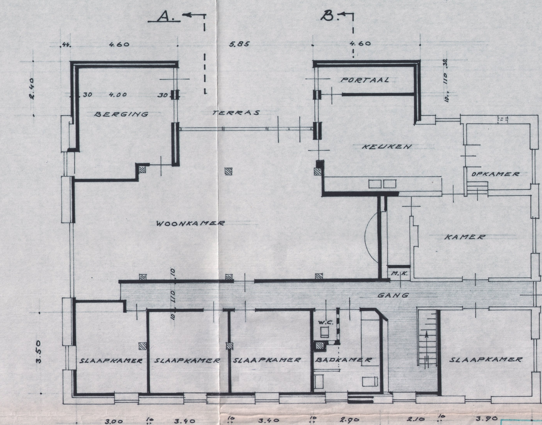
- BEGANEGROND -
