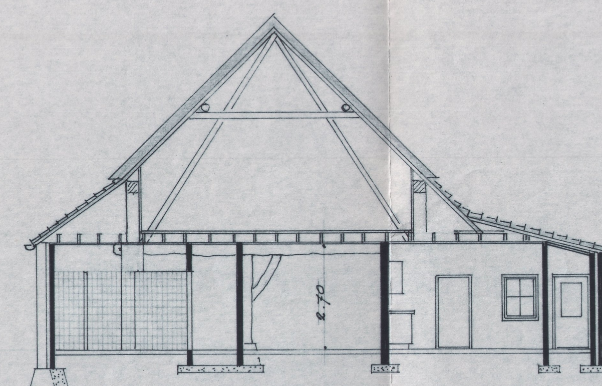
- DOORSNEDEN - B -
