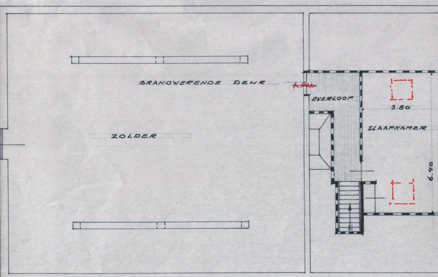
- VERDIEPING -
