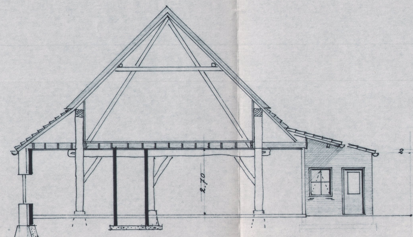
- DOORSNEDEN - A -
