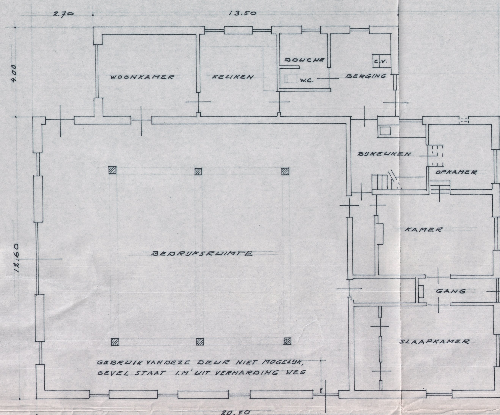
- BESTAANDE - BEGANEGROND -
