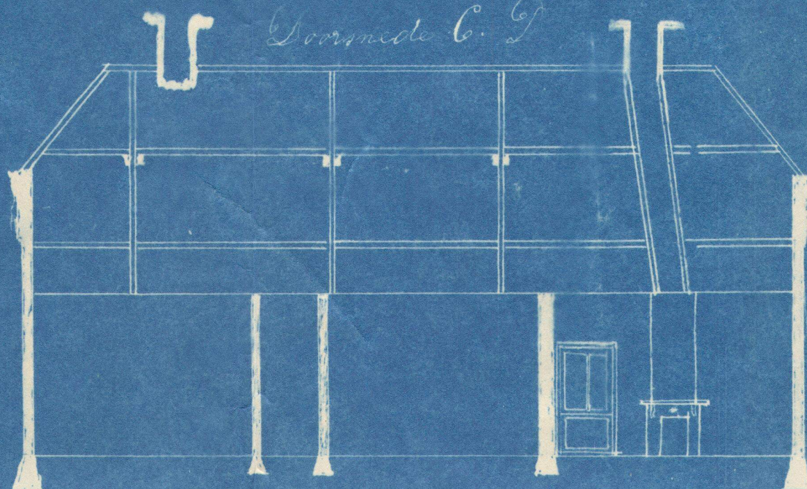
Doorsnede A. B.
