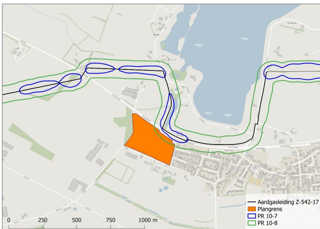
Figuur 2. Plaatsgebonden risicocontouren aardgasbuisleiding 5.1.2e
