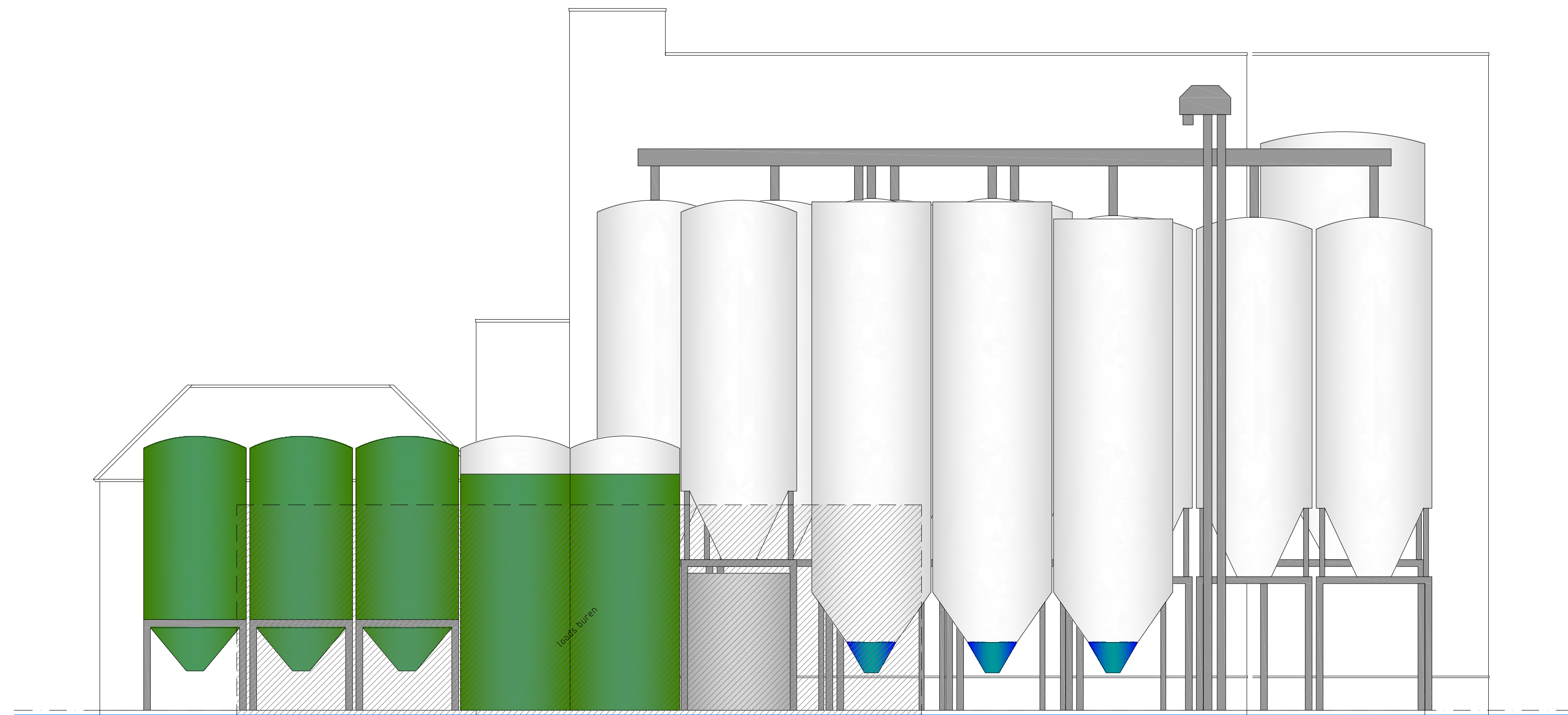
ZIJ AANZICHT - NIEUW 1:100
