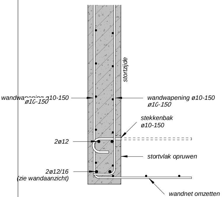
Stekkenbak aansluiting
