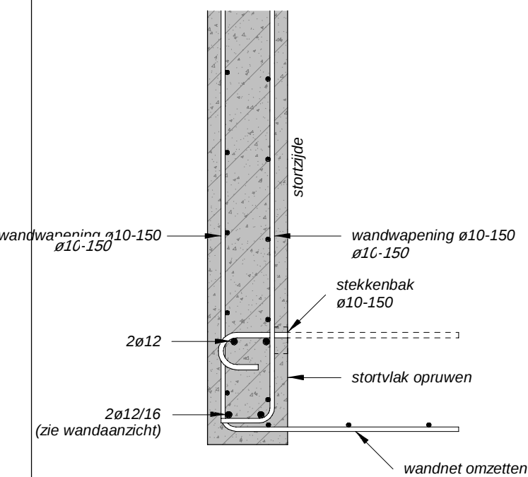
Stekkenbak aansluiting
