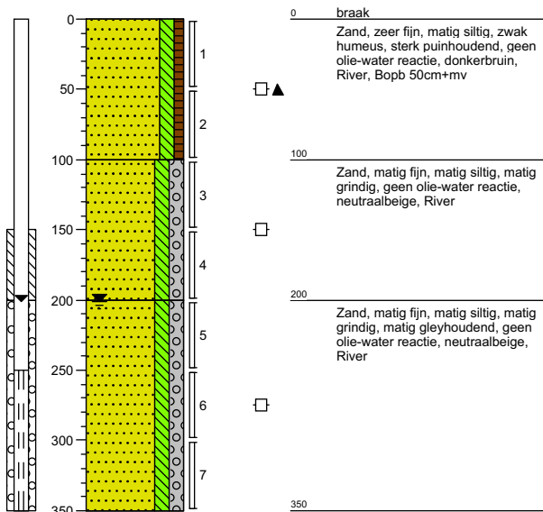
Boring: C03
