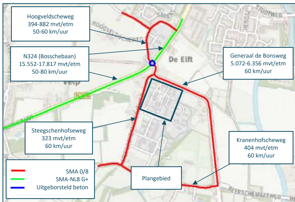
Figuur 3 Verkeers- en verhardingsgegevens lokale wegen 2035
