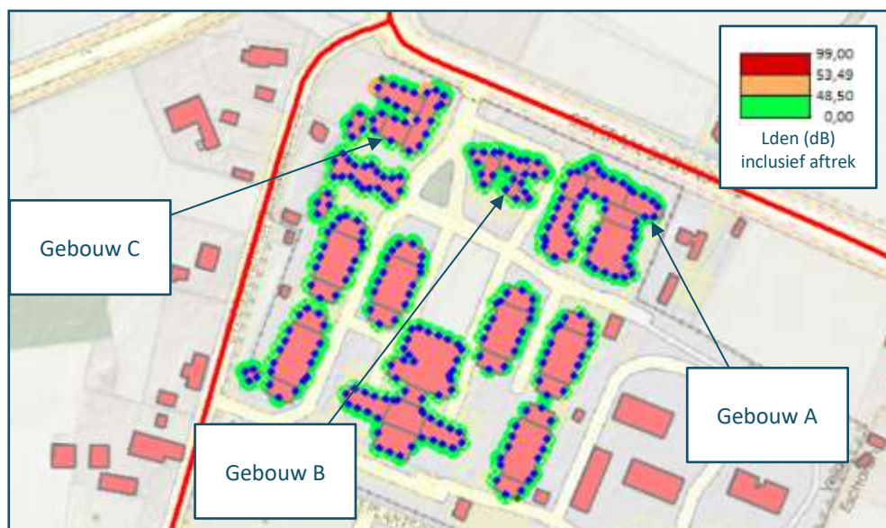
Figuur 6 Geluidsbelasting op het plangebied vanwege wegverkeer op de N324 met overschrijdingen van de voorkeursgrenswaarde (oranje).
