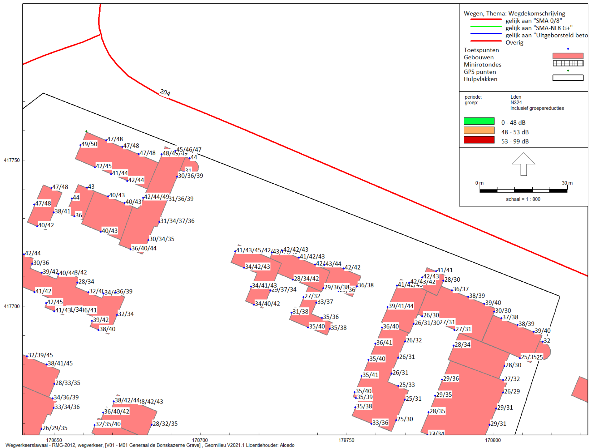
Figuur 7 Rekenresultaten van wege wegverkeer op de N324 op de noordzijde van het plangebied inclusief 5 dB aftrek
