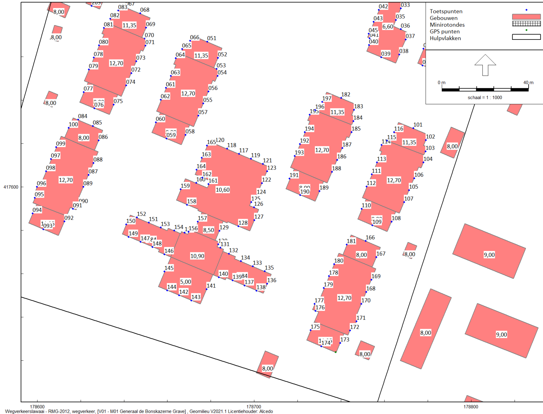
Figuur 5 Ligging en nummering toetspunten zuidzijde plangebied
