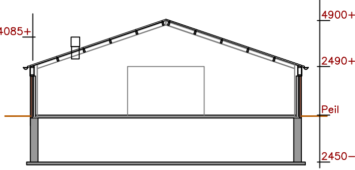
Doorsnede B-B 1:200
