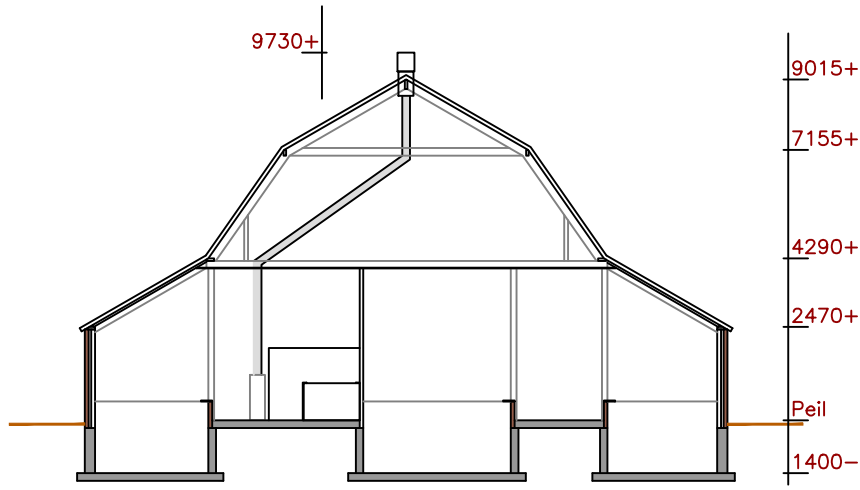
Doorsnede A-A 1:200
