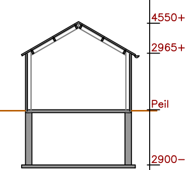
Doorsnede E-E 1:200
