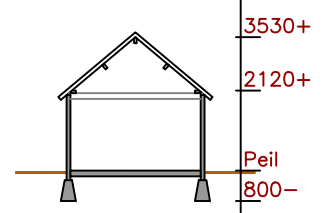
Doorsnede D-D 1:200
