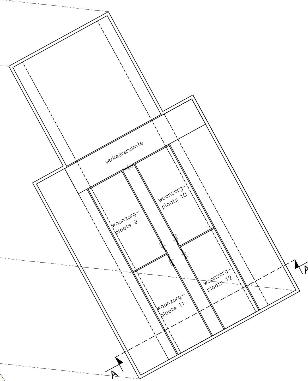
Eerste verdieping
