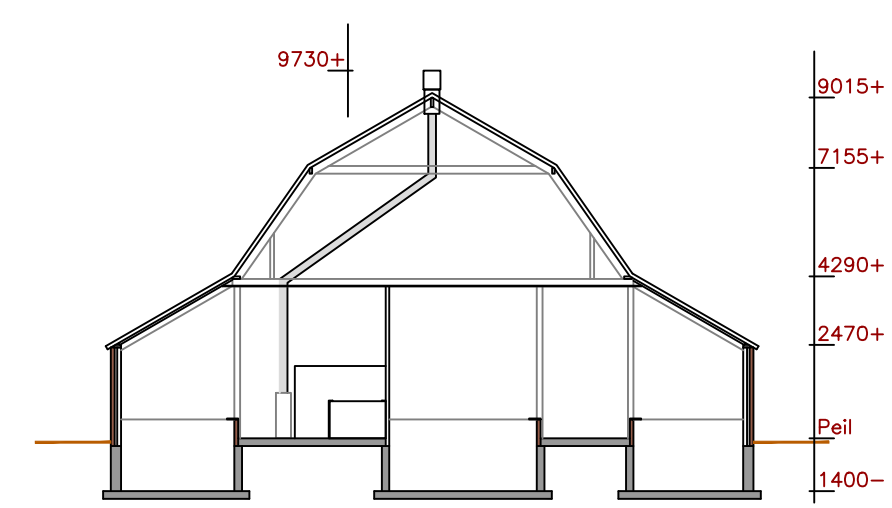
Doorsnede A-A 1:200
