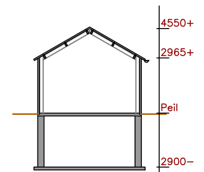
Doorsnede E-E 1:200
