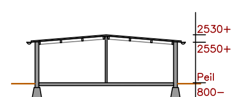
Doorsnede F-F 1:200
