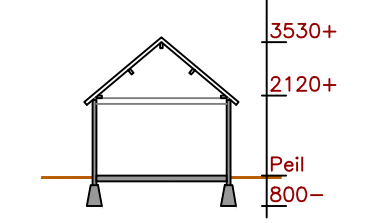
Doorsnede D-D 1:200
