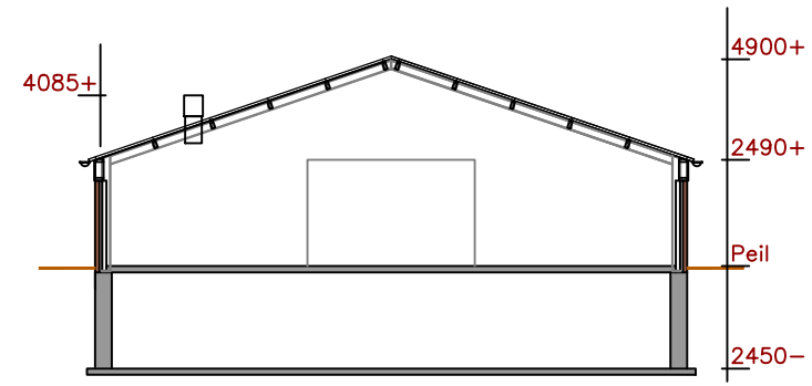
Doorsnede B-B 1:200
