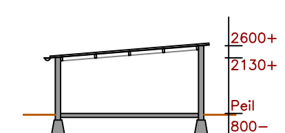
Doorsnede G-G 1:200
